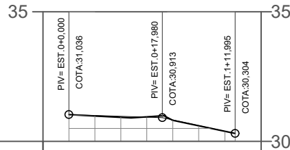
PERFIL EIXO DA RUA SDO 82
