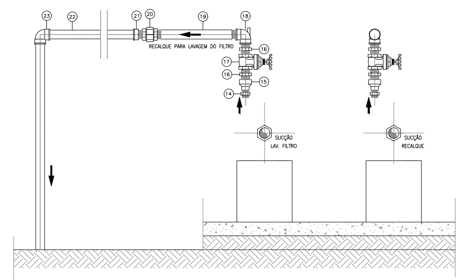
07 ELEVACÃO ESCALA 1/10
