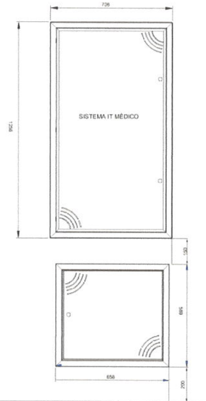
← Imagem ilustrativa de quatro Sistemas IT Médico em centro de distribuição embutido SIT14000/DT-E e SIT14000/TE.
