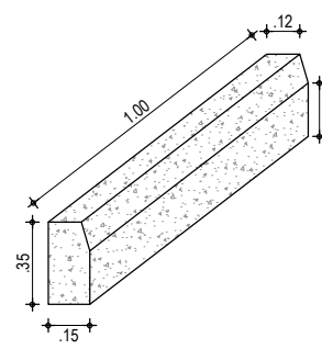
03 DETALHE DO MEIO FIO ESCALA SEM
