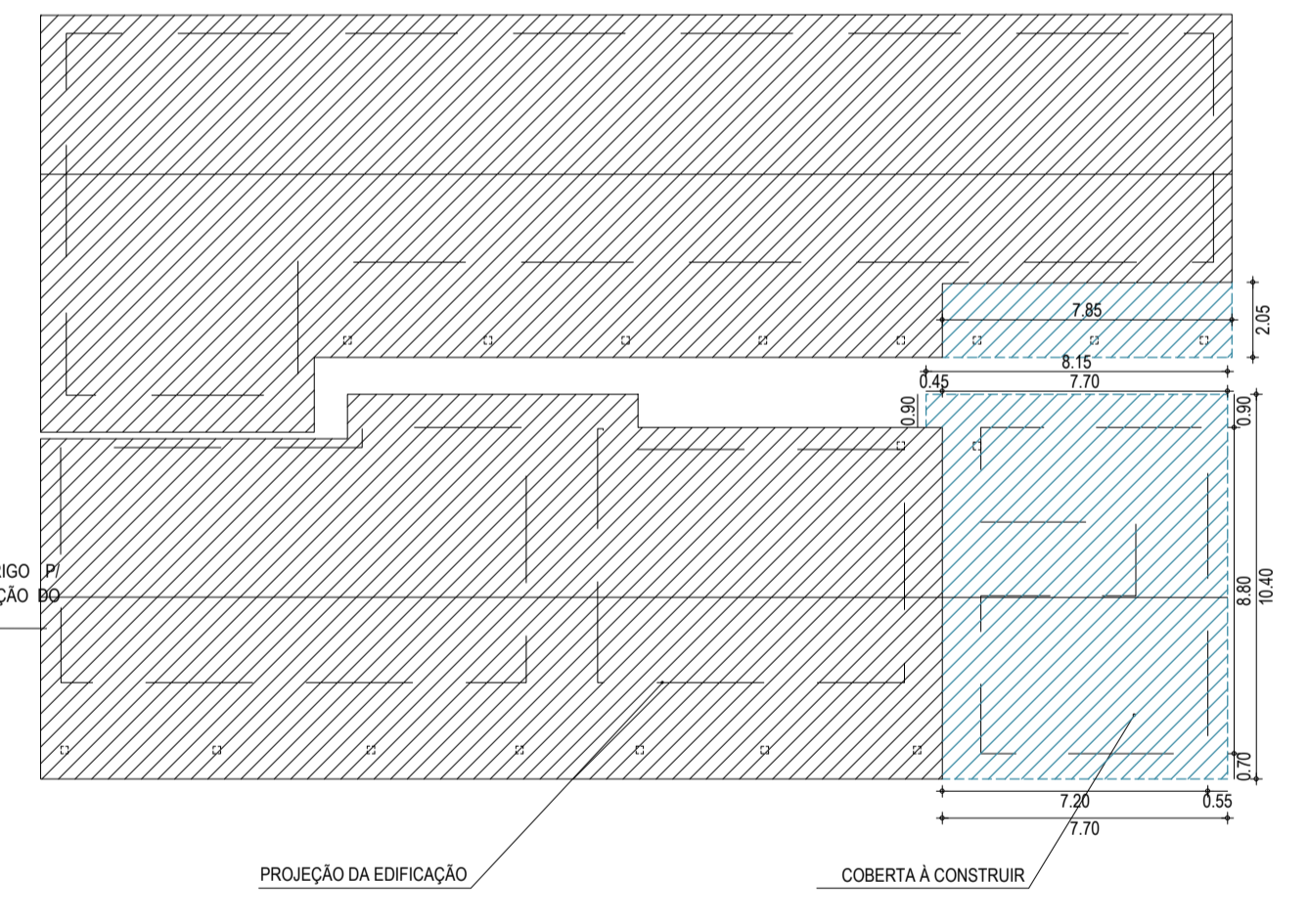
02 PLANTA DE REFORMA | COBERTA ESCALA: 1/200
