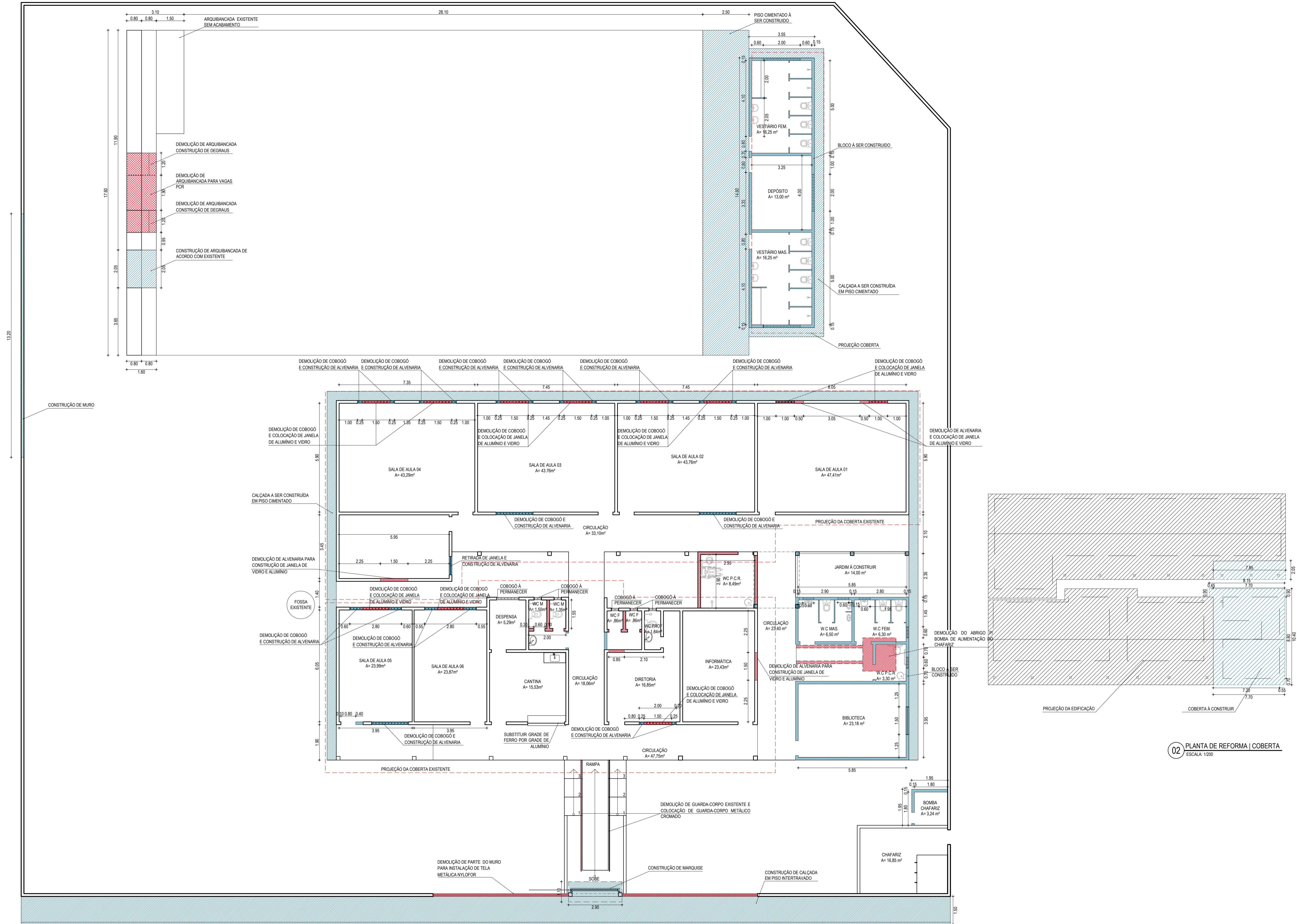
01 PLANTA DE REFORMA | EDIFICAÇÃO ESCALA: 1/100
