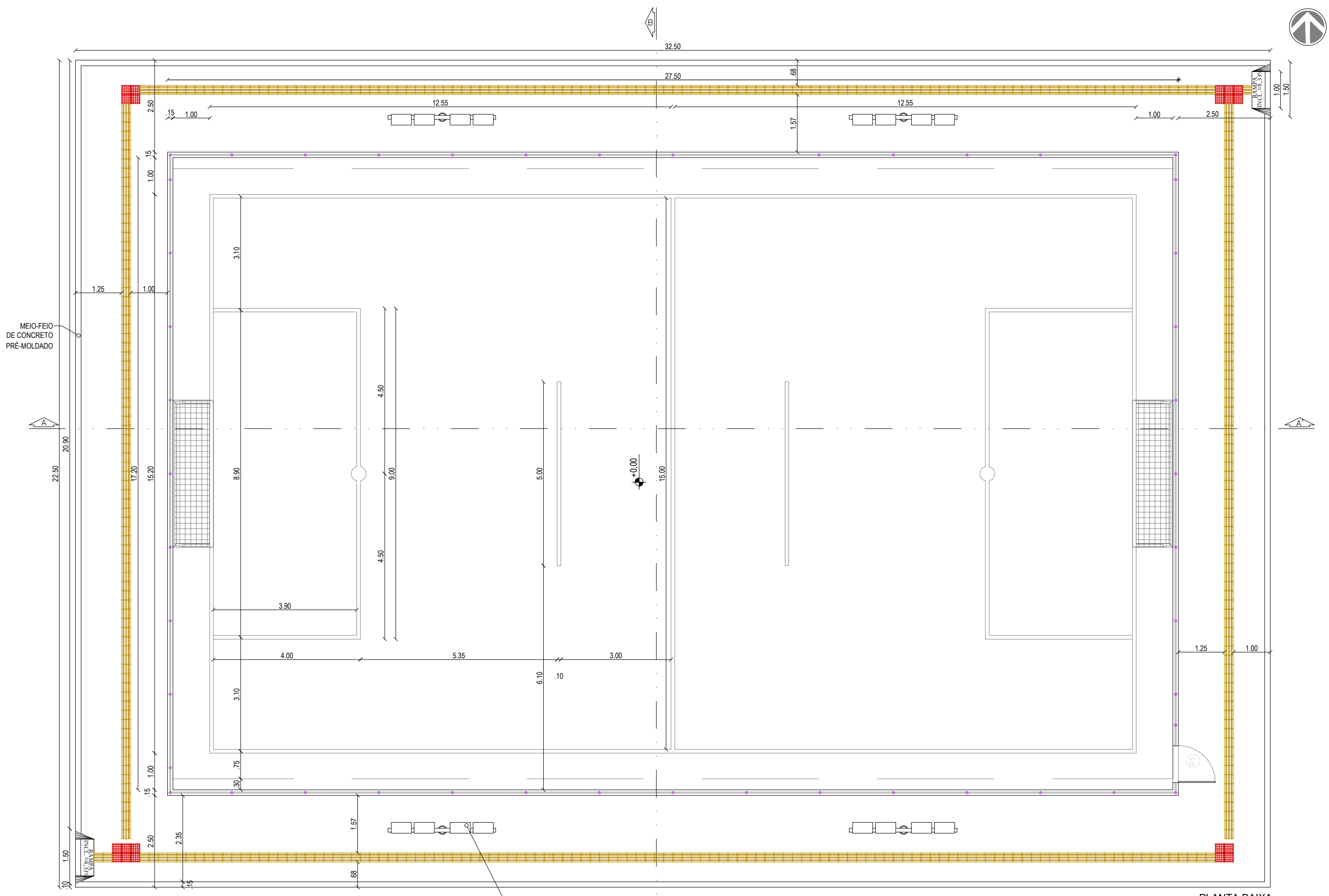
1 PLANTA BAIXA esc.: 1/100
