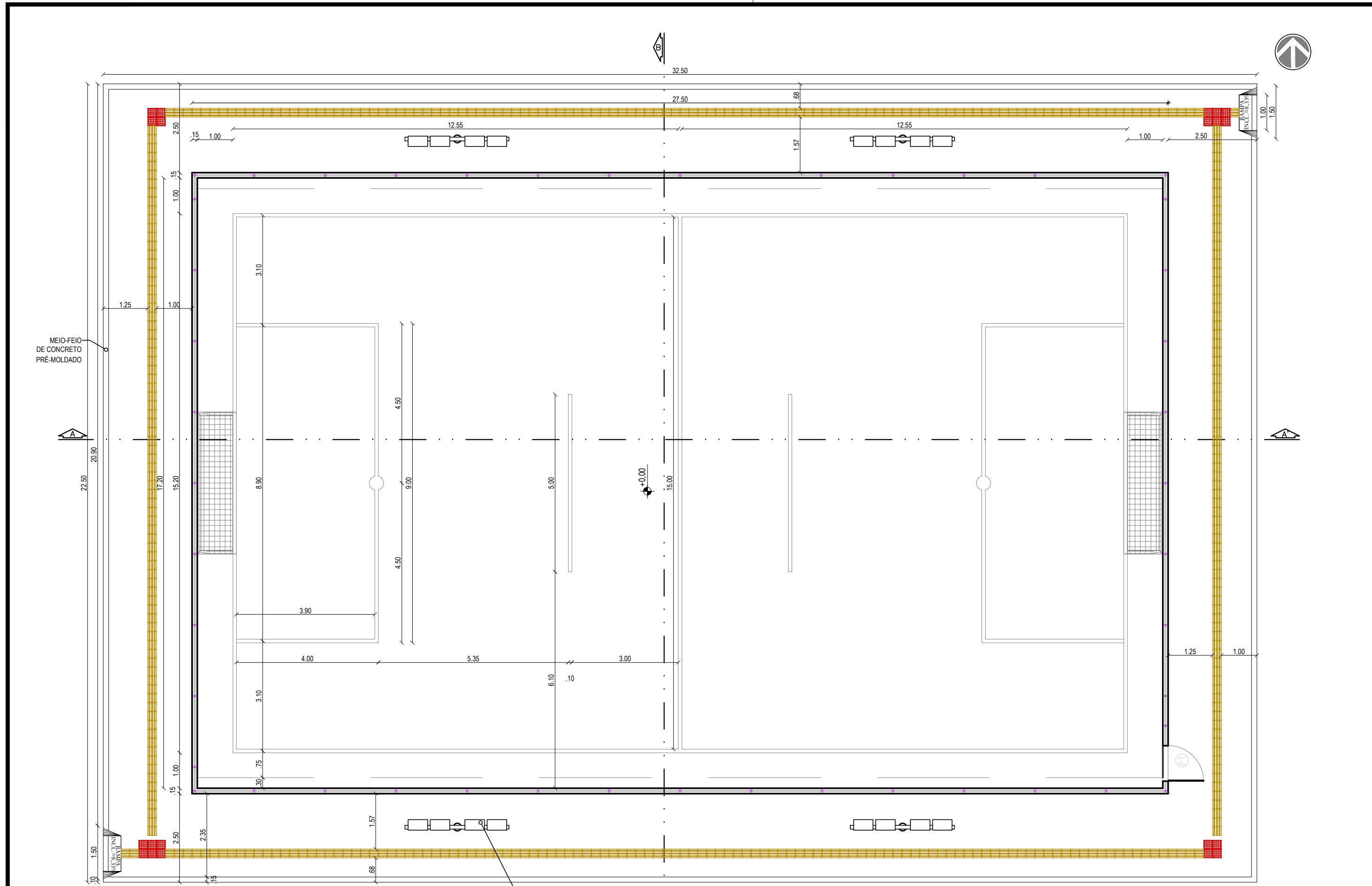
1 PLANTA BAIXA esc.: 1/100
