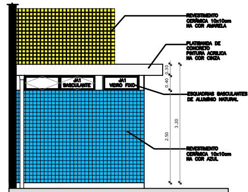
VESTIÁRIO: VISTA G- FACHADA LATERAL
