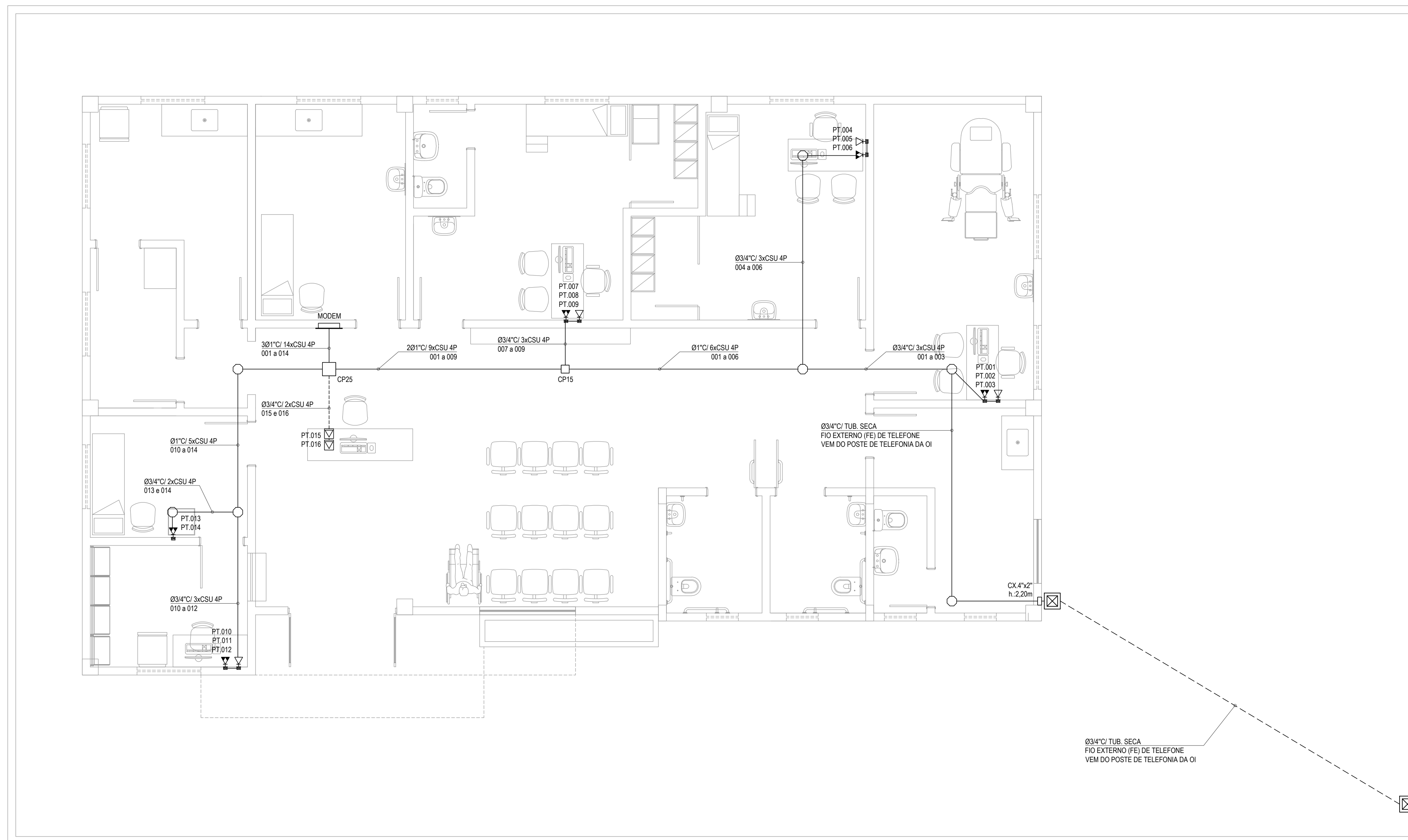
PLANTA BAIXA - TELECOMUNICAÇÕES ESCALA: 1/50
