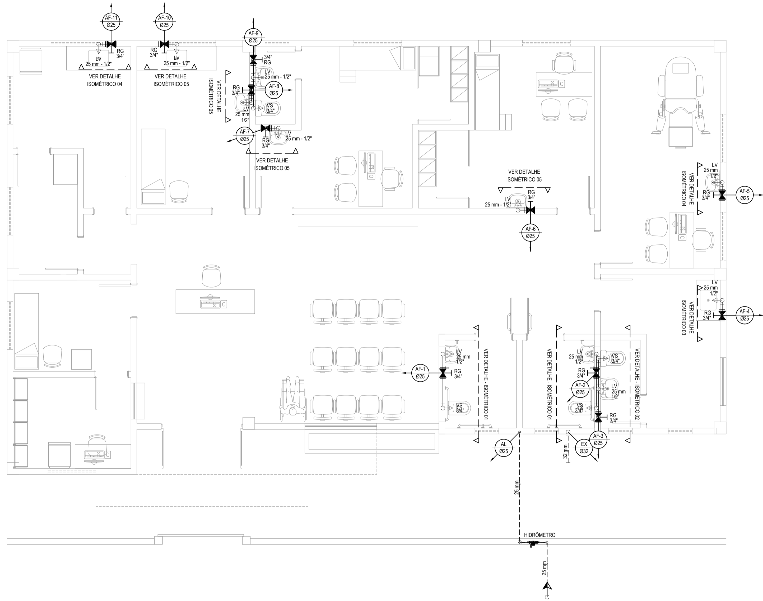
TÉRREO - INSTALAÇÕES HIDRÁULICAS ESCALA: 1/50
