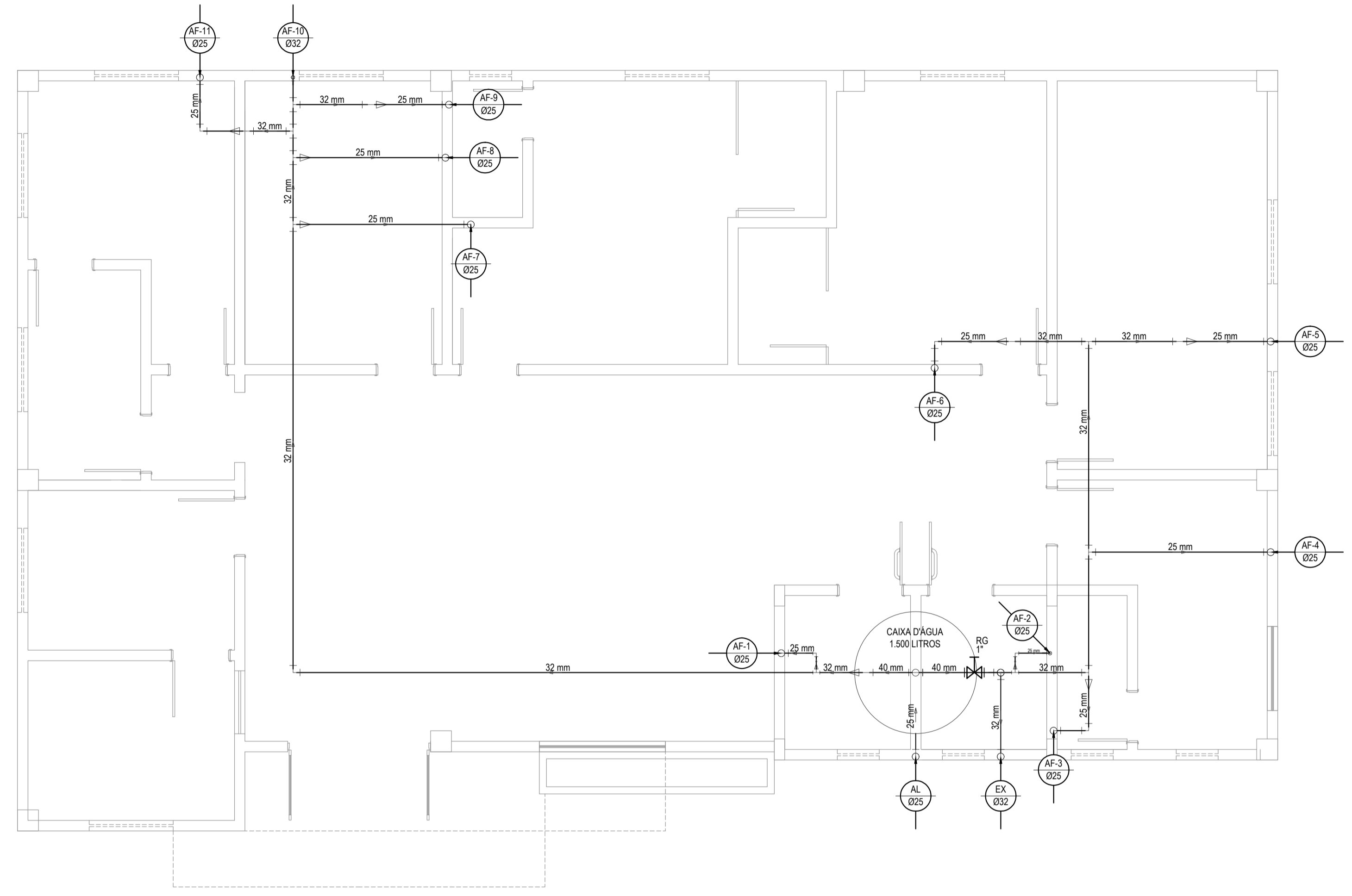
COBERTA - INSTALAÇÕES HIDRÁULICAS ESCALA: 1/50
