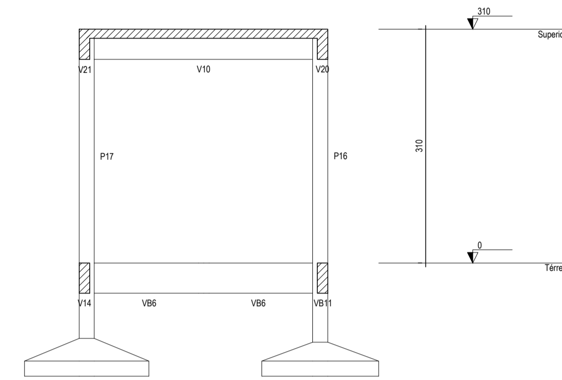
04 CORTE D-D ESCALA: 1:50
