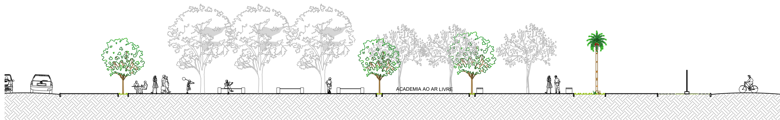
01 CORTE AA ESCALA 1/200
