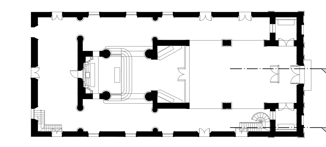
03 PLANTA INDICATIVA DE CORTE ESC. 1/250
