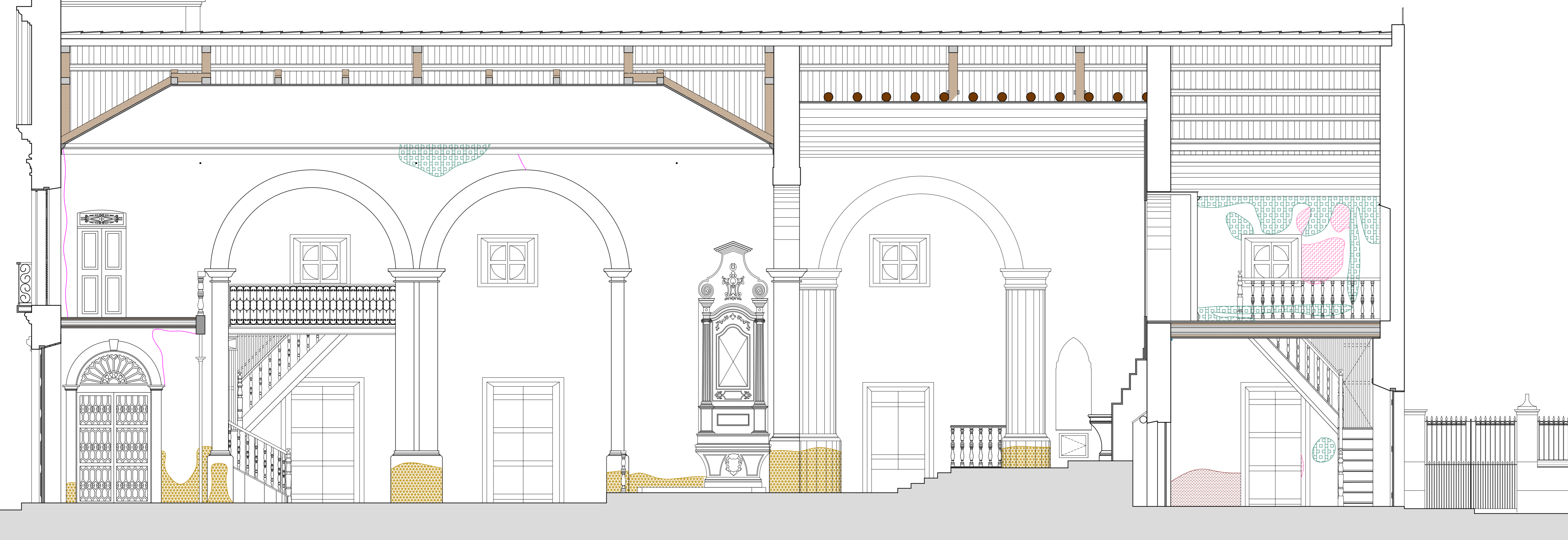
02 CORTE M ESC. 1/50
