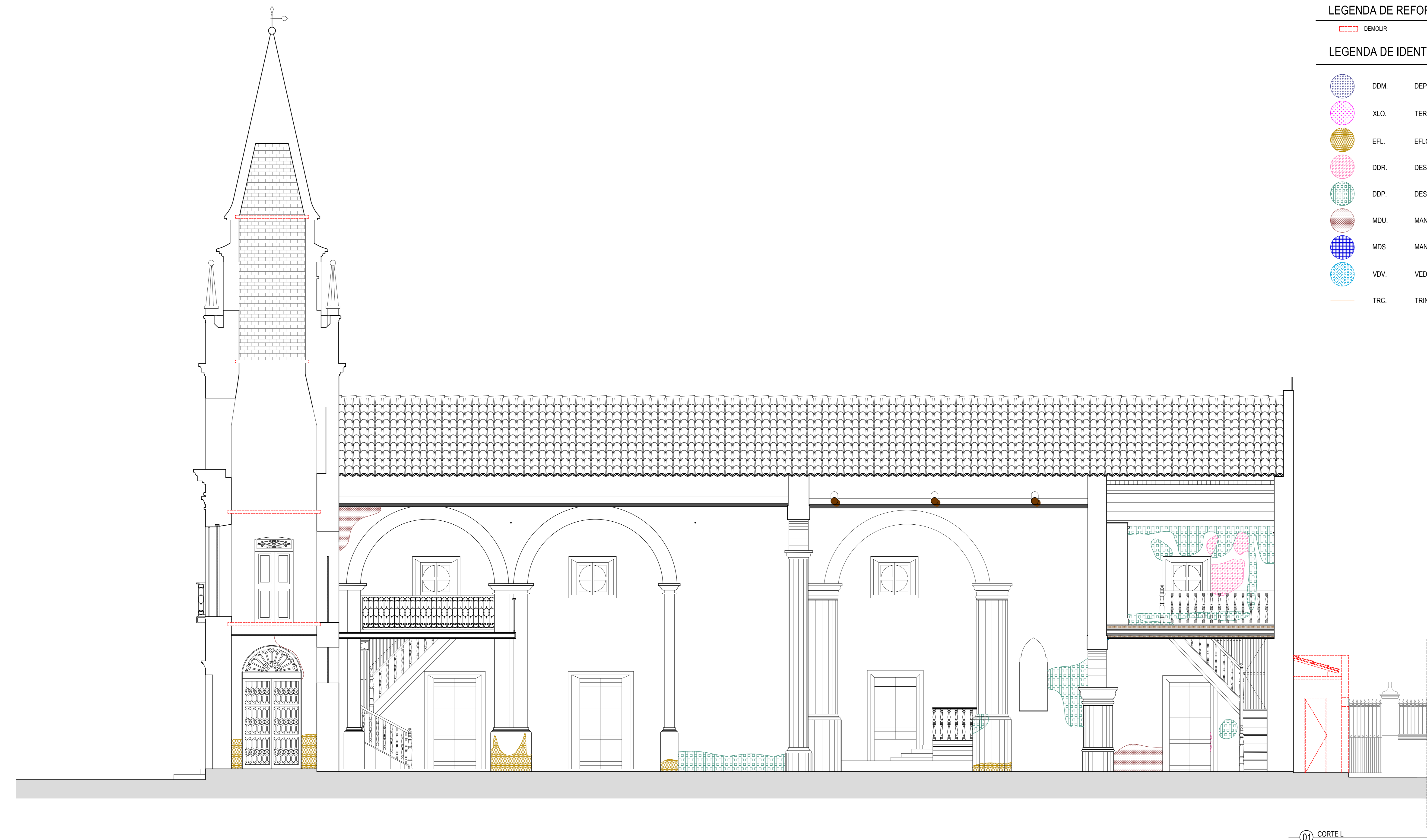
01 CORTE L ESC. 1/50
