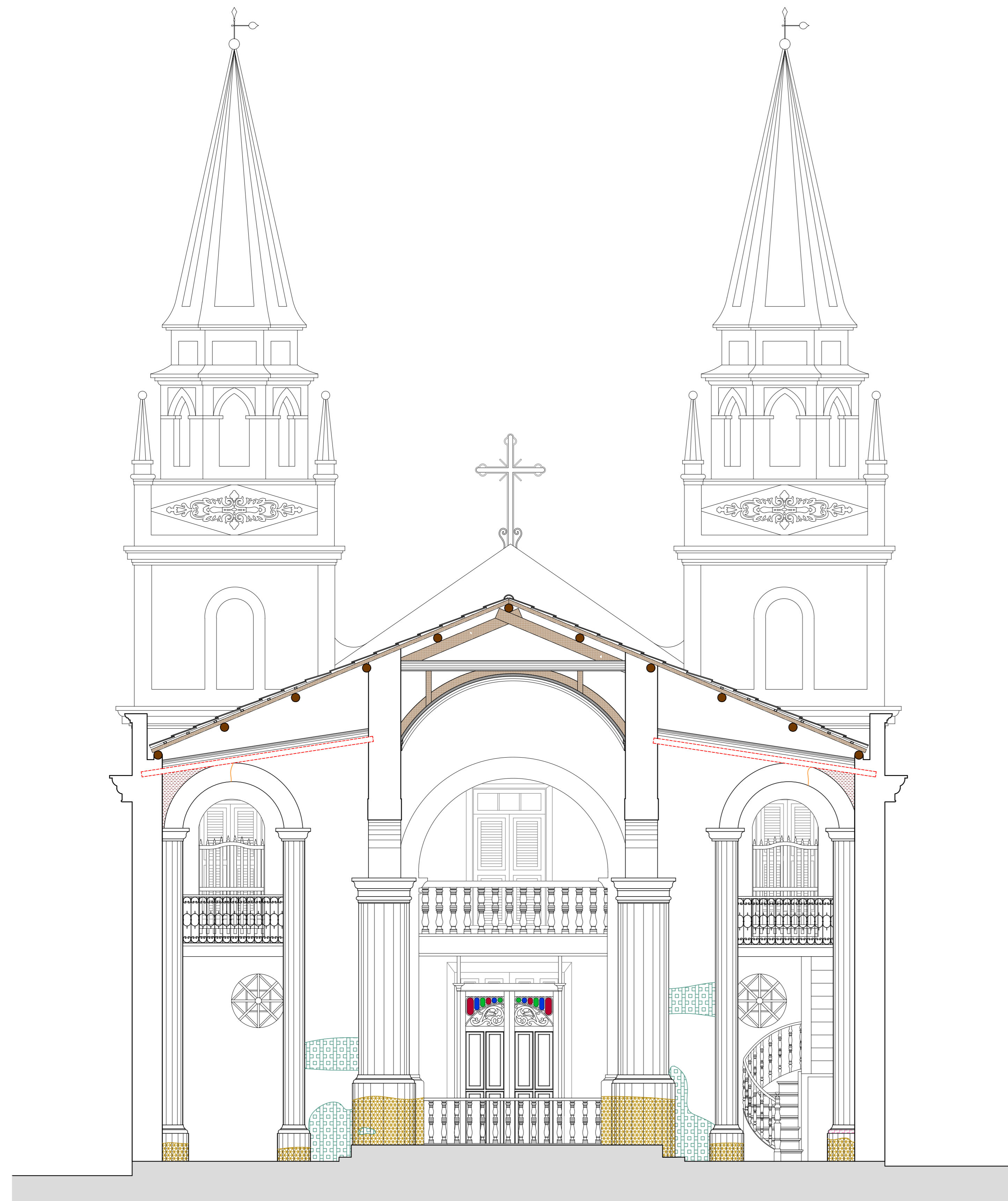
01 CORTE F ESC.: 1/50
