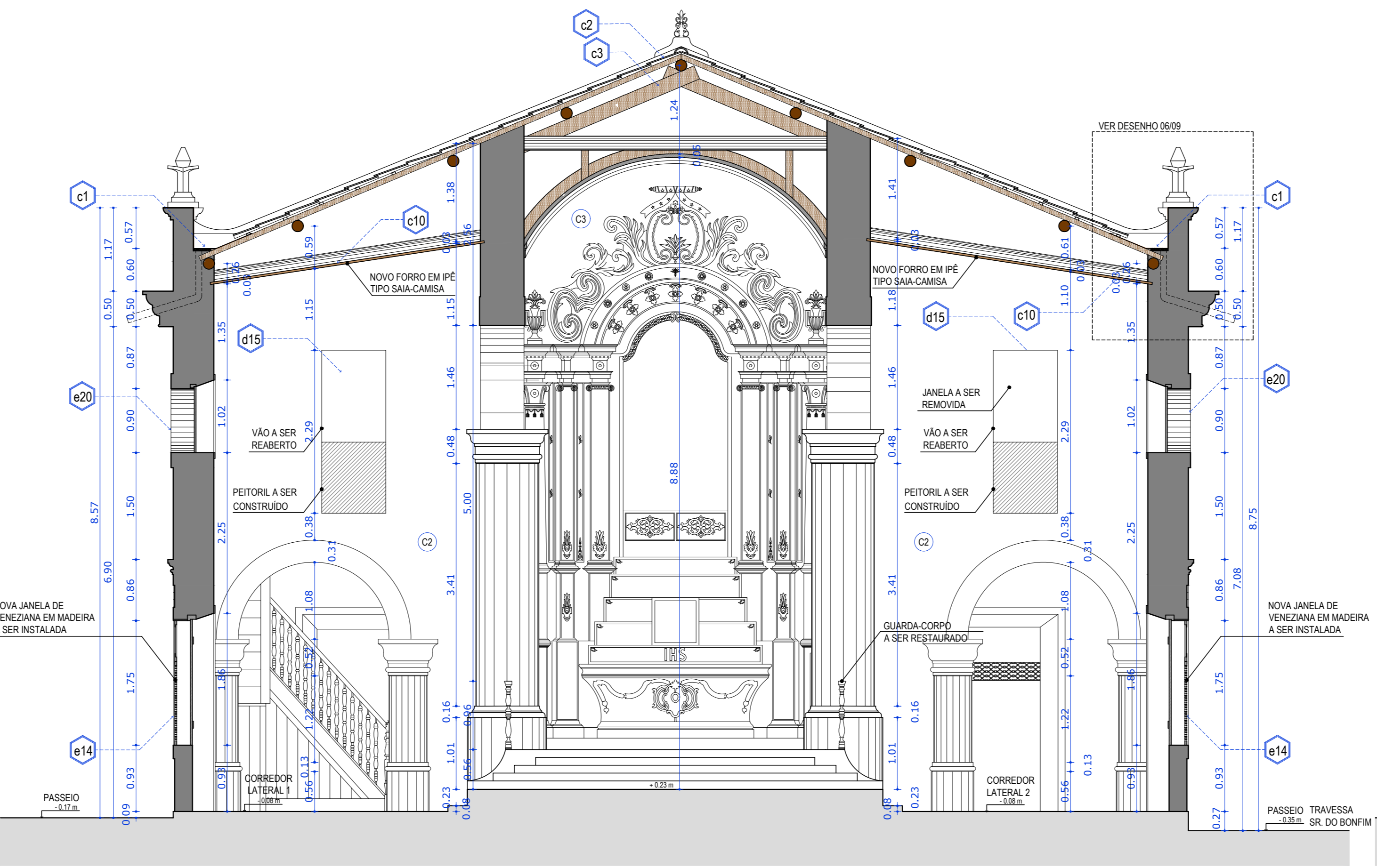
02 CORTE B - CONSTRUÇÃO ESC. 1/50
