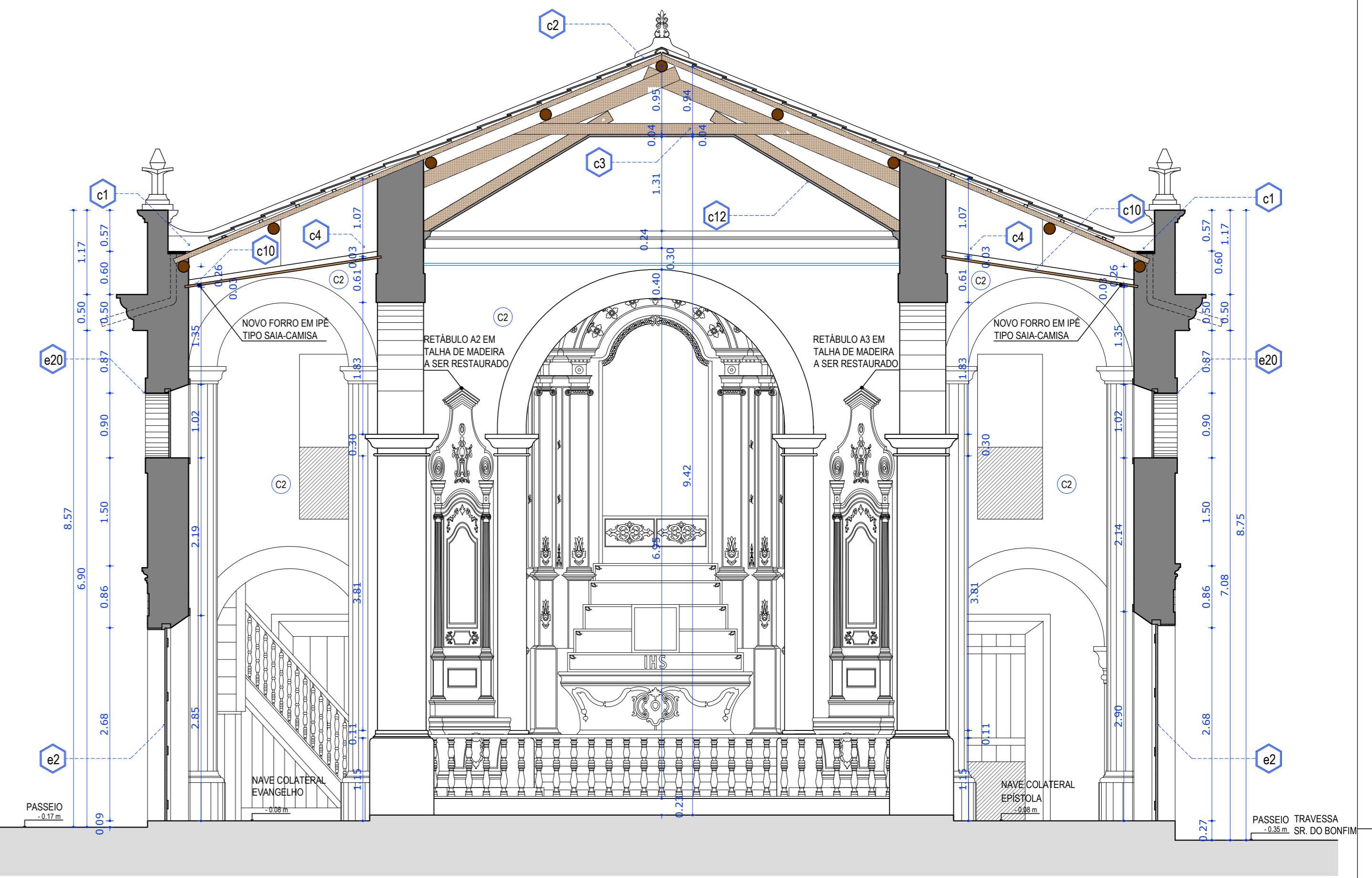
03 CORTE C - CONSTRUÇÃO ESC. 1/50
