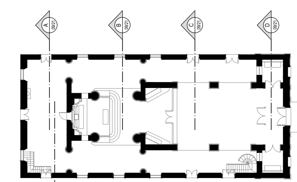
08 PLANTA INDICATIVA DE CORTE ESC. 1/250
