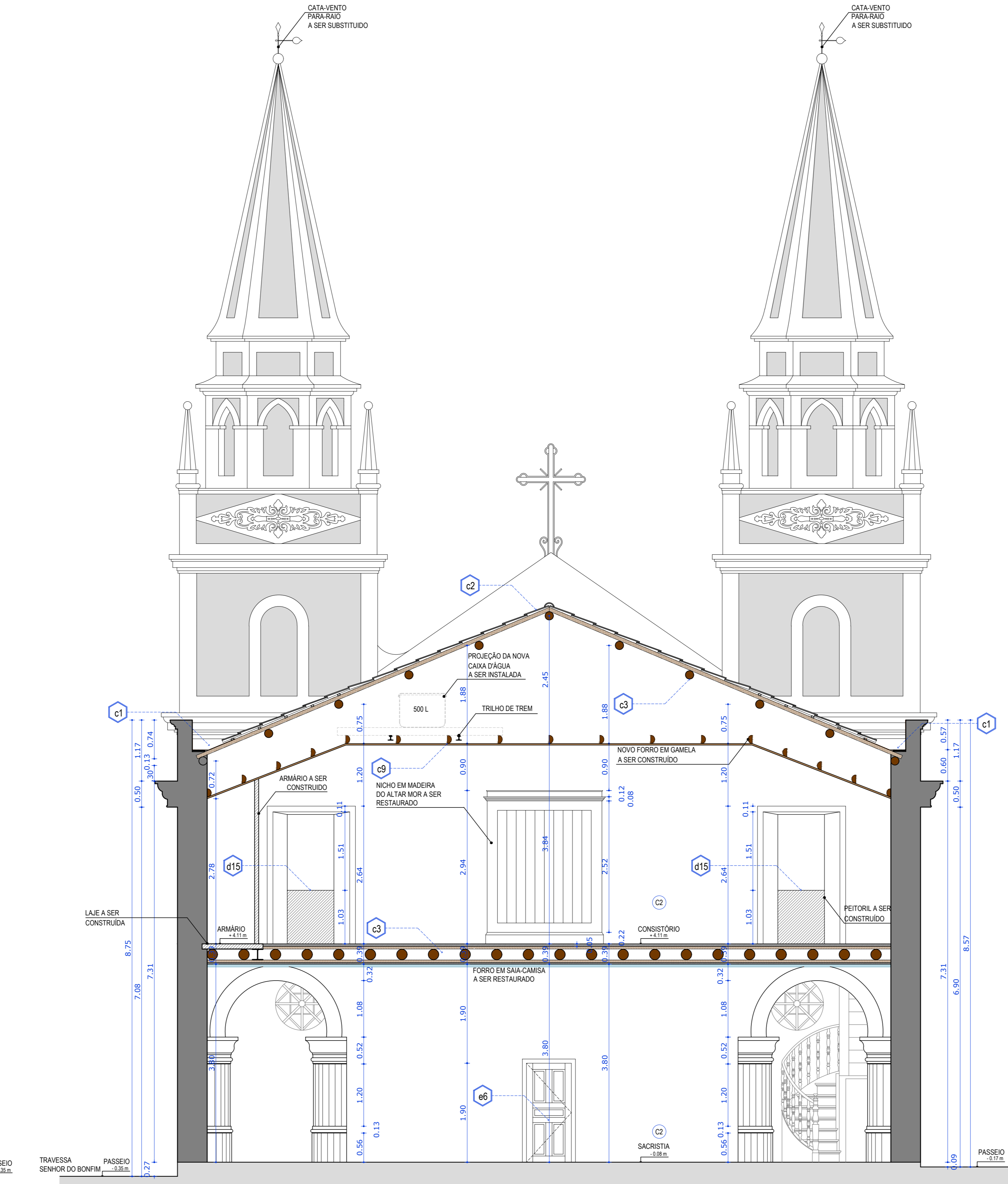
05 CORTE E - CONSTRUÇÃO ESC. 1/50
