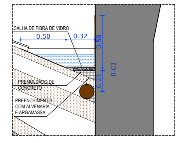
07 DETALHE 2 DA NOVA CALHA ESC. 1/20
