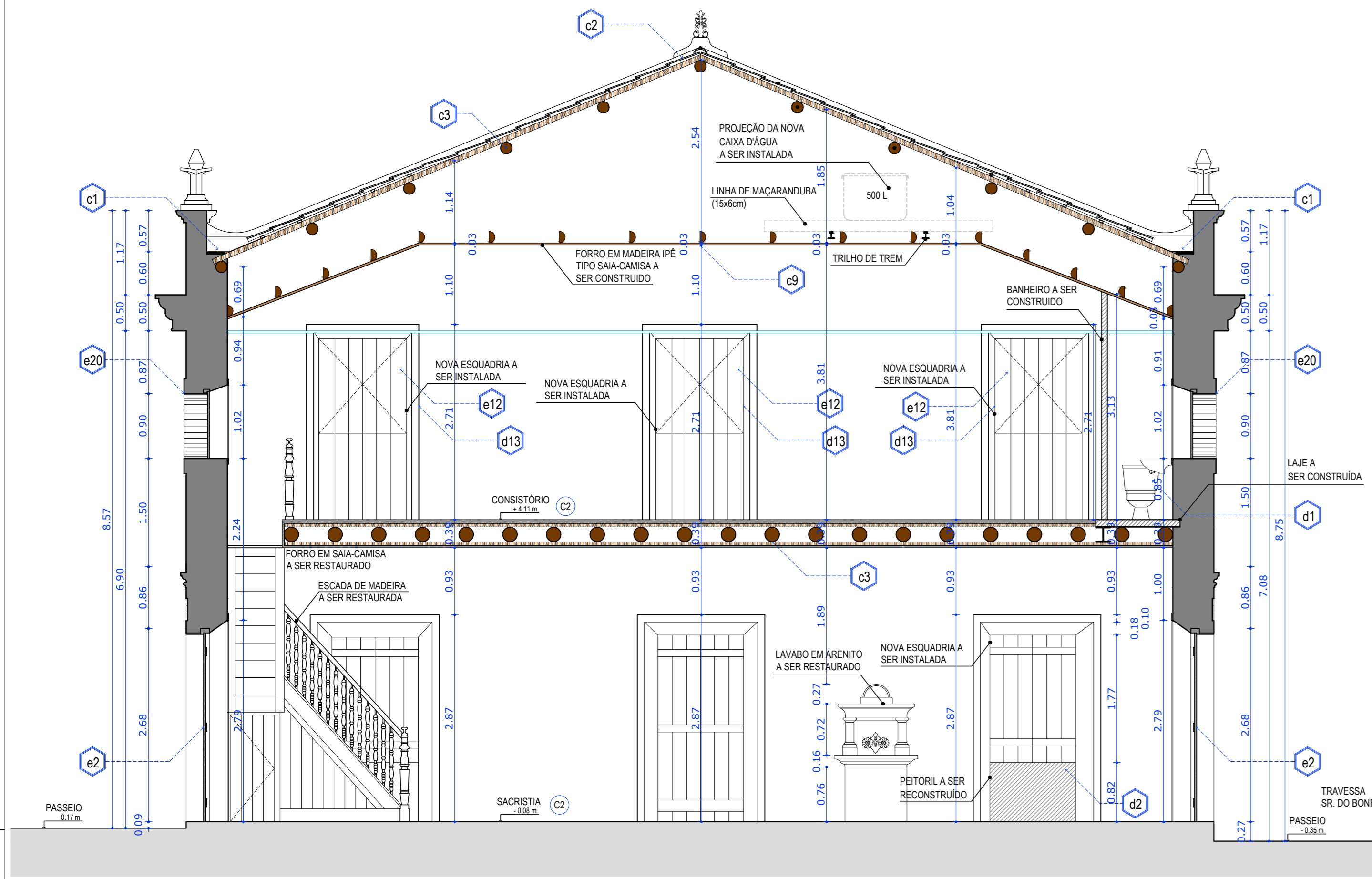
01 CORTE A - CONSTRUÇÃO ESC. 1/50
