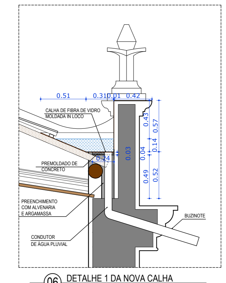
06 DETALHE 1 DA NOVA CALHA ESC. 1/20
