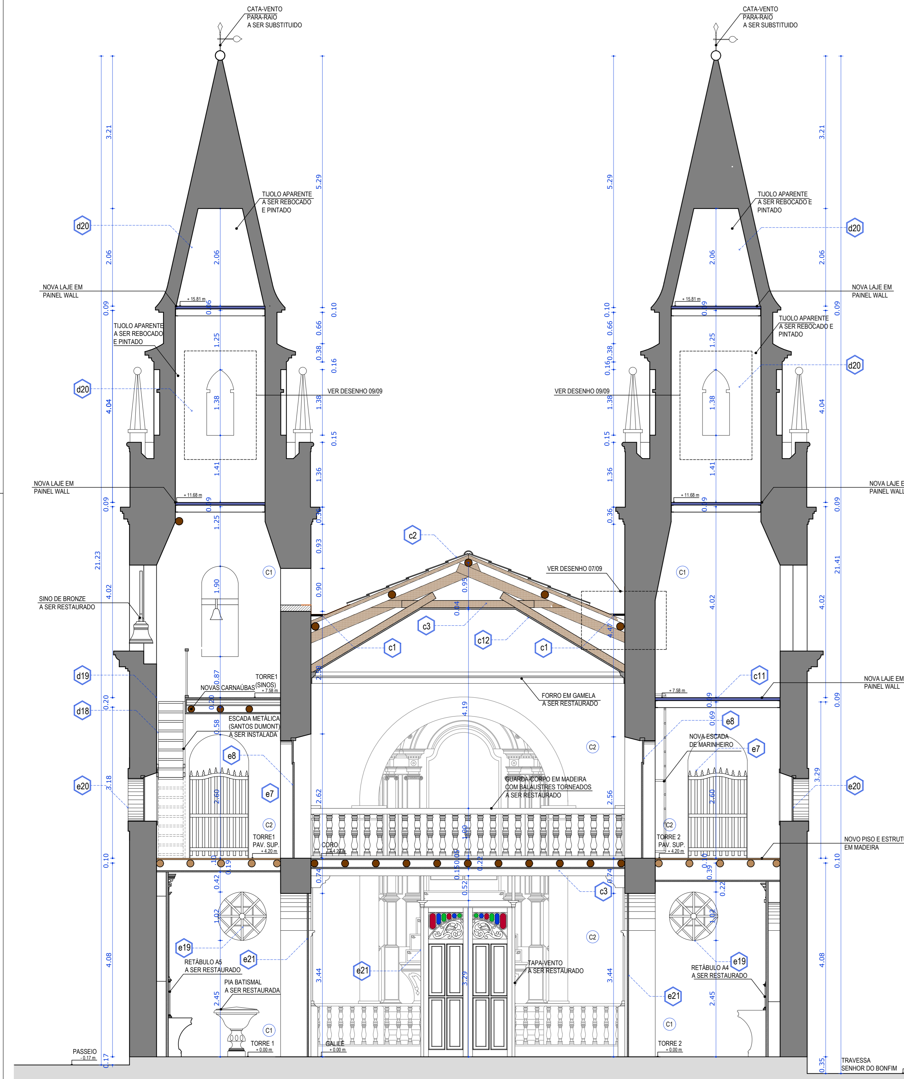
04 CORTE D - CONSTRUÇÃO ESC. 1/50
