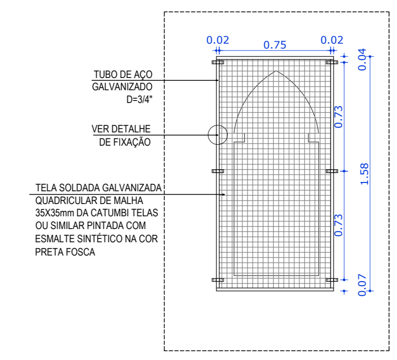
08 DETALHE DA TELA METÁLICA ESC. 1/20
