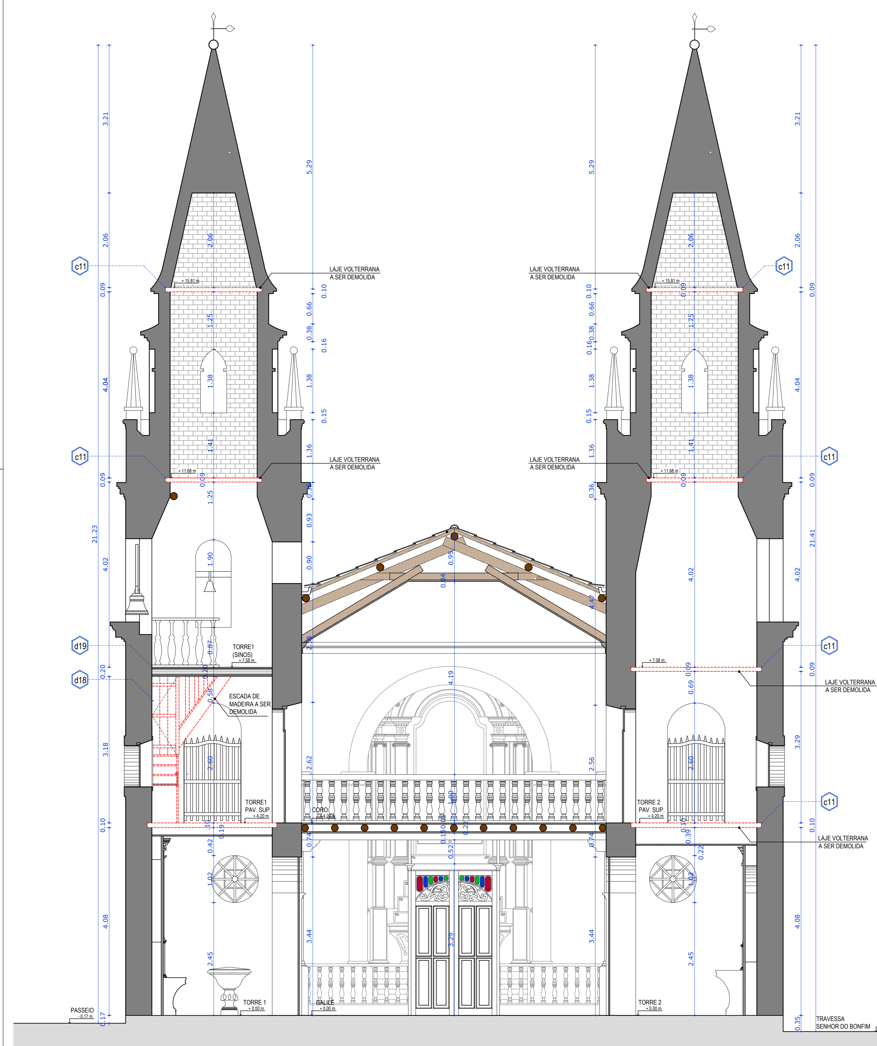
04 CORTE D - DEMOLIÇÃO ESC. 1/50
