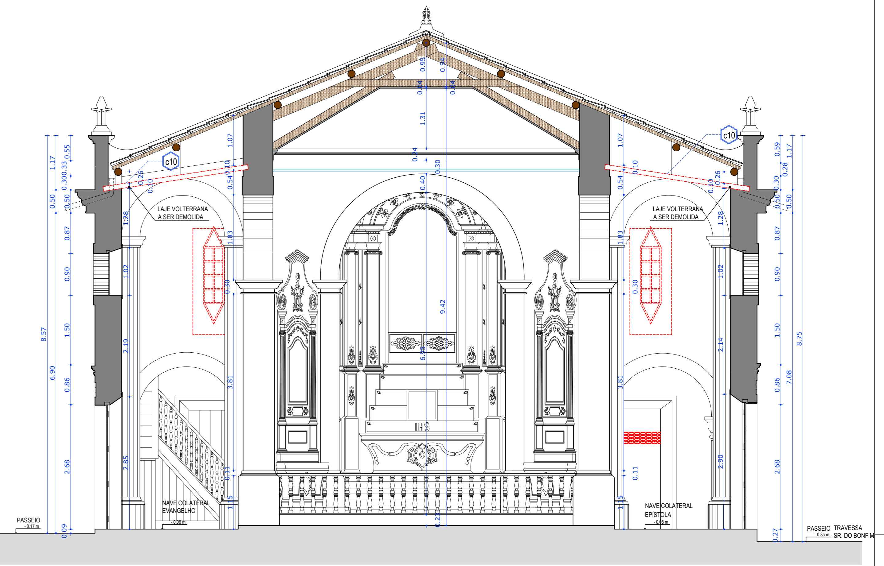
03 CORTE C - DEMOLIÇÃO ESC. 1/50
