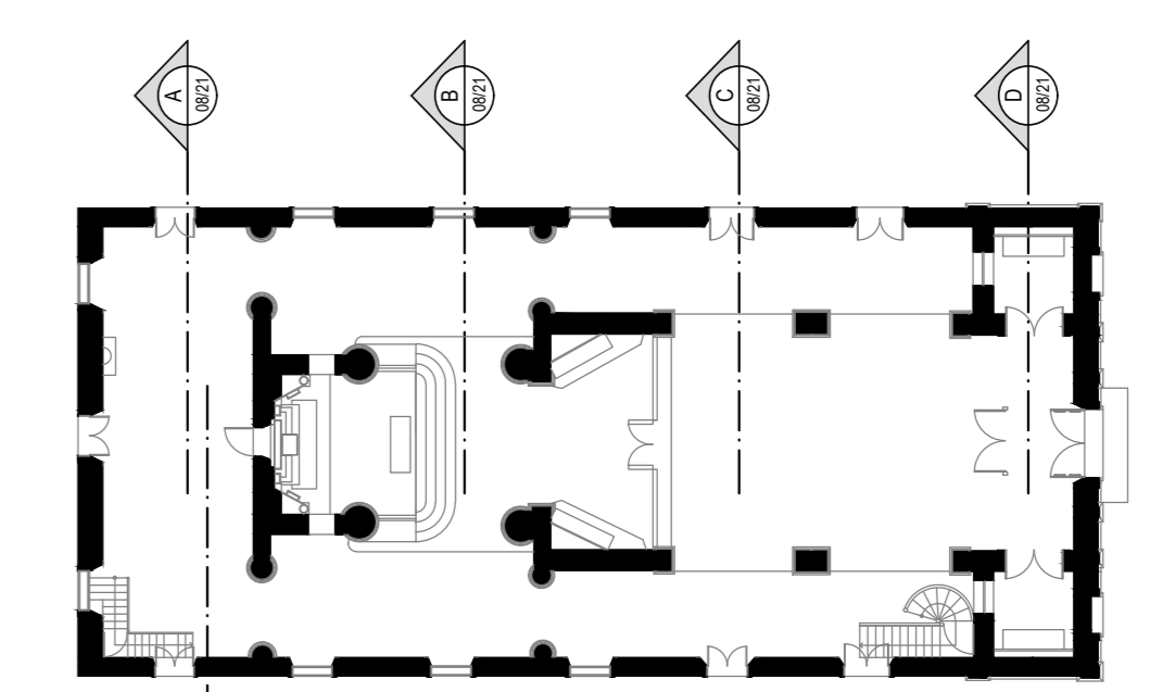
06 PLANTA INDICATIVA DE CORTE ESC. 1/200
