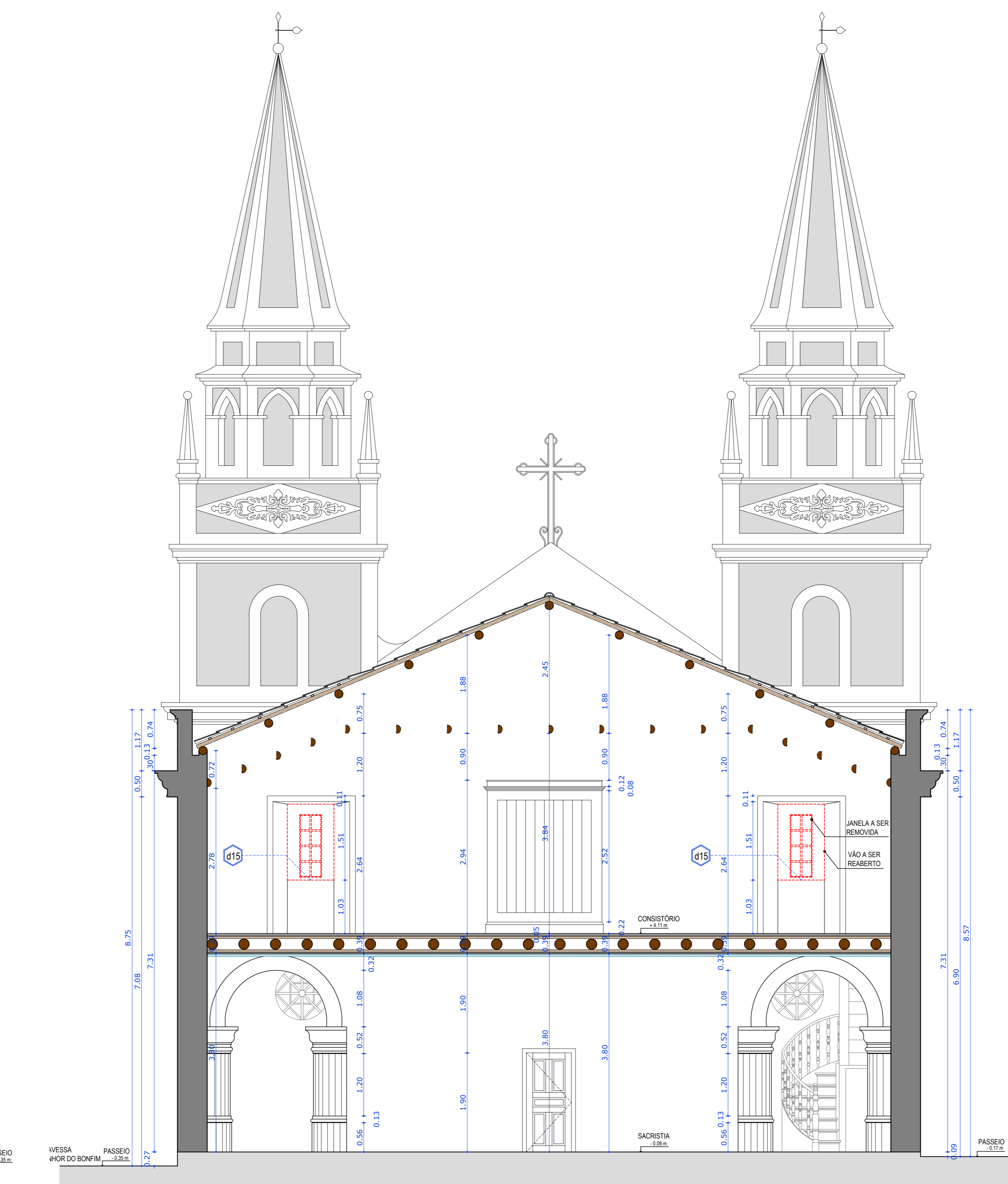
05 CORTE E - DEMOLIÇÃO ESC. 1/50
