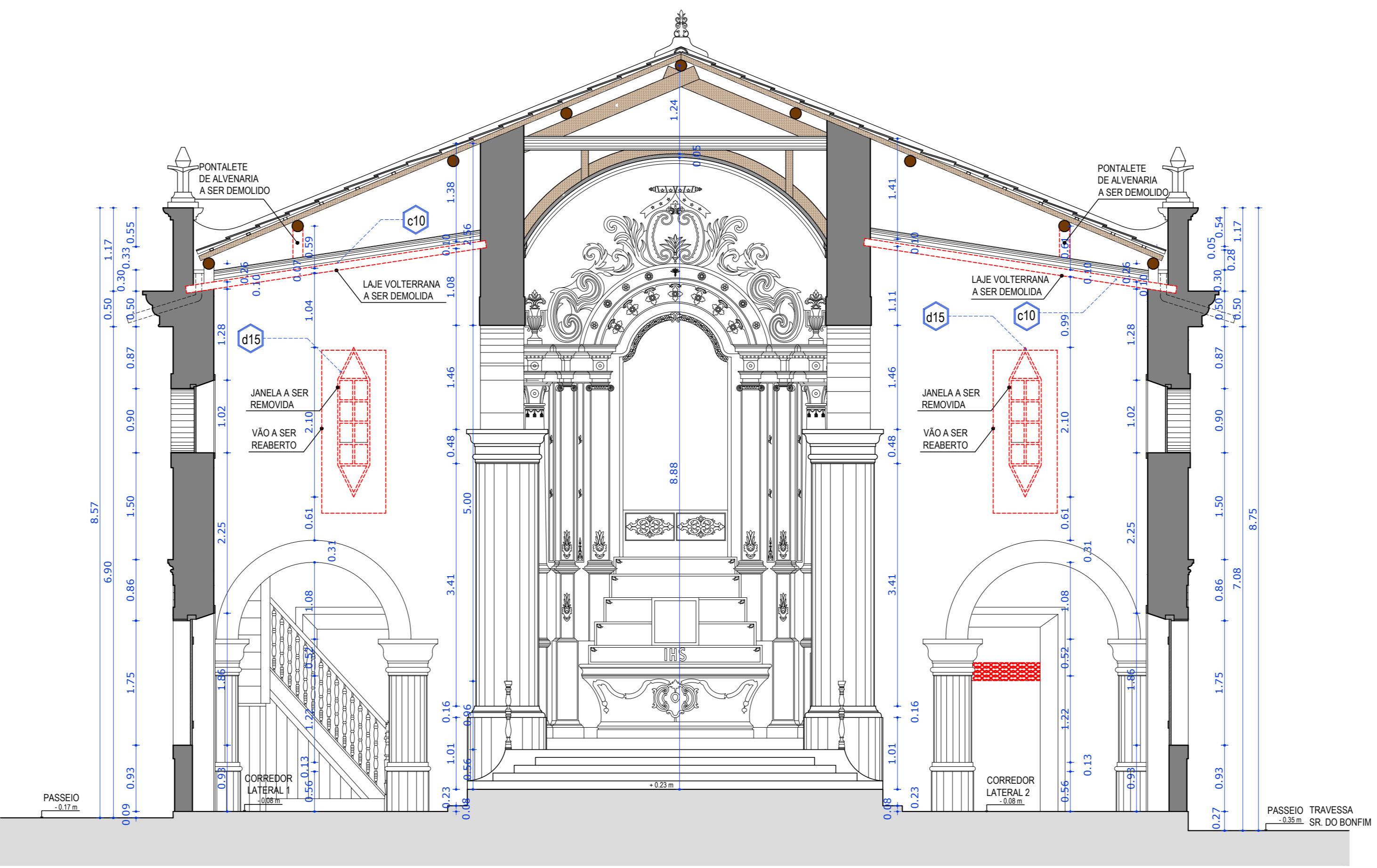
02 CORTE B - DEMOLIÇÃO ESC. 1/50
