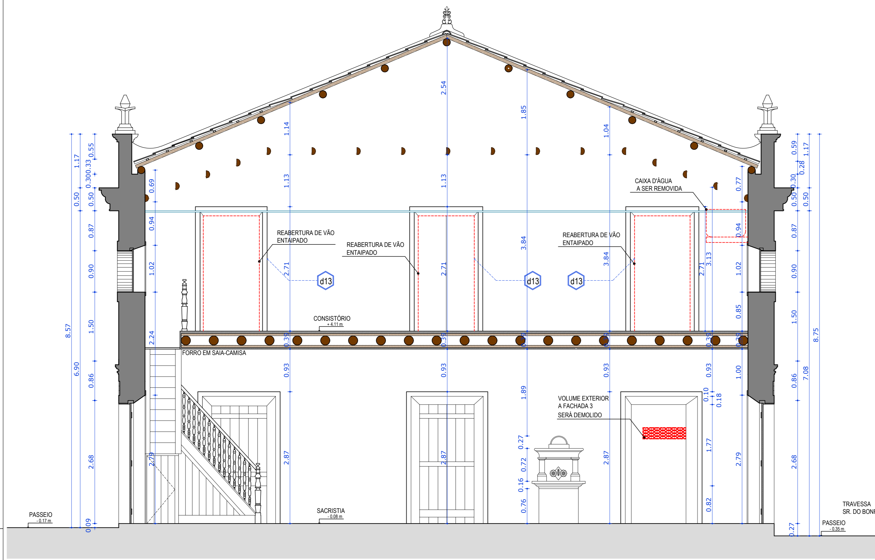
01 CORTE A - DEMOLIÇÃO ESC. 1/50
