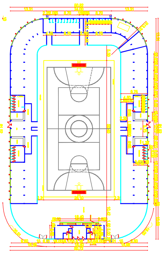
01.00 PLANTA BAIXA ALVENARIA
