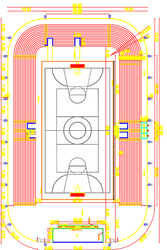
01.01 PLANTA BAIXA ARQUIBANCADA
