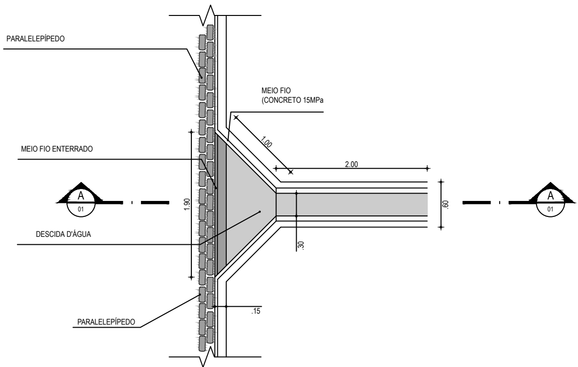
01 DETALHE SAÍDA D'ÁGUA ESCALA 1/50
