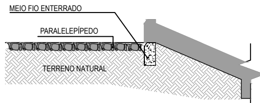
02 CORTE AA ESCALA 1/50
