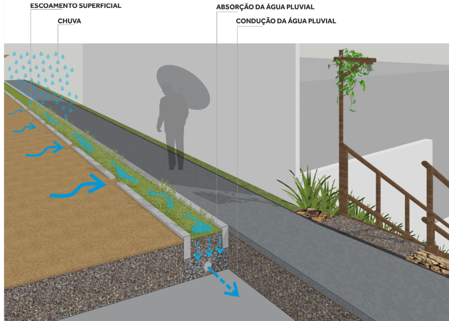
PERSPECTIVA - BIOVALETA sem escala
