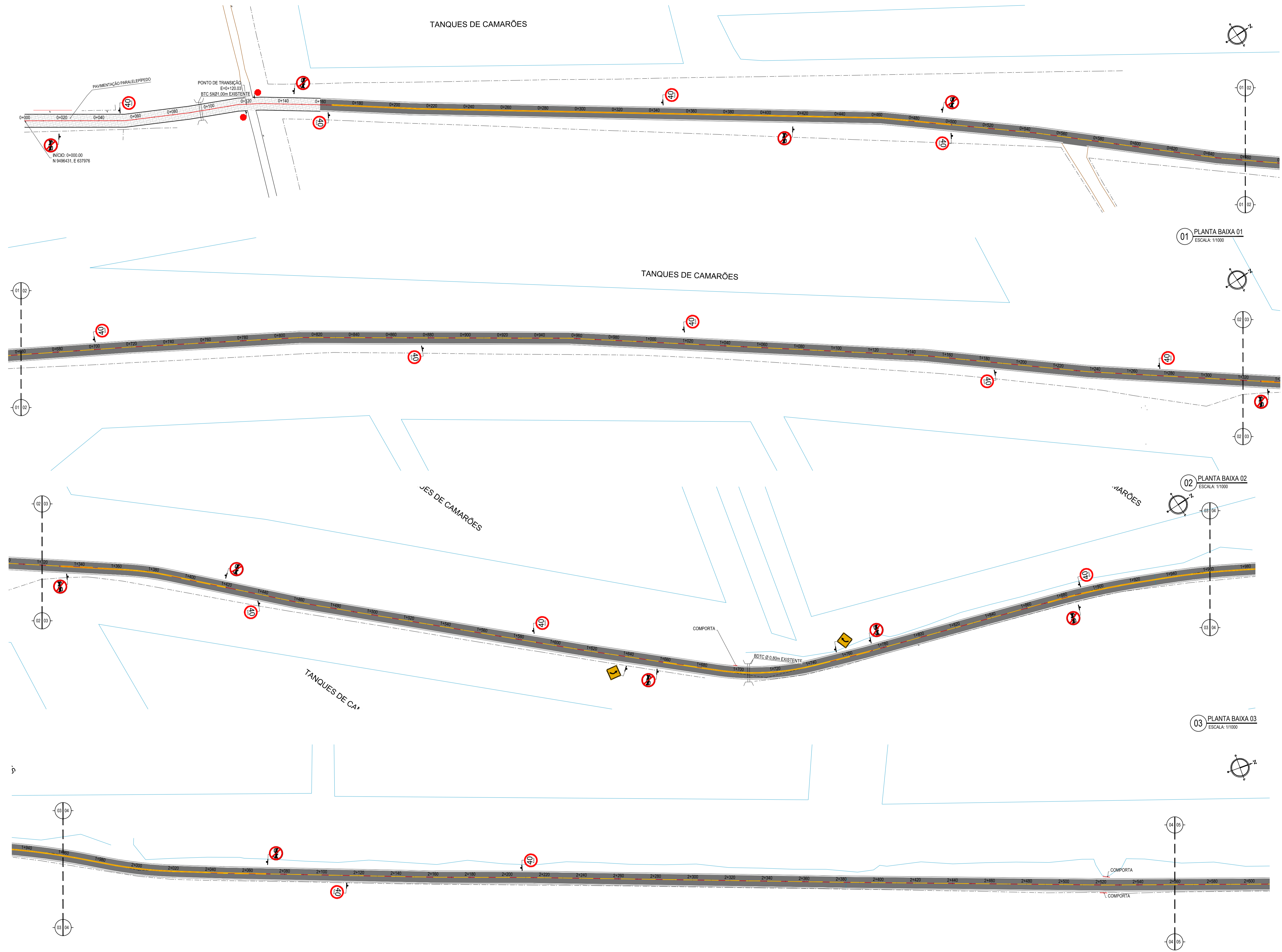
04 PLANTA BAIXA 04 ESCALA: 1/1000
