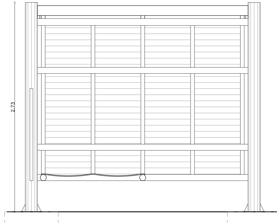
VISTA 01 esc 1:25
