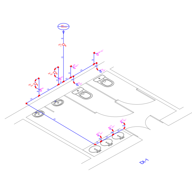
DETALHE, DI-1 ESC _____ 1/50
