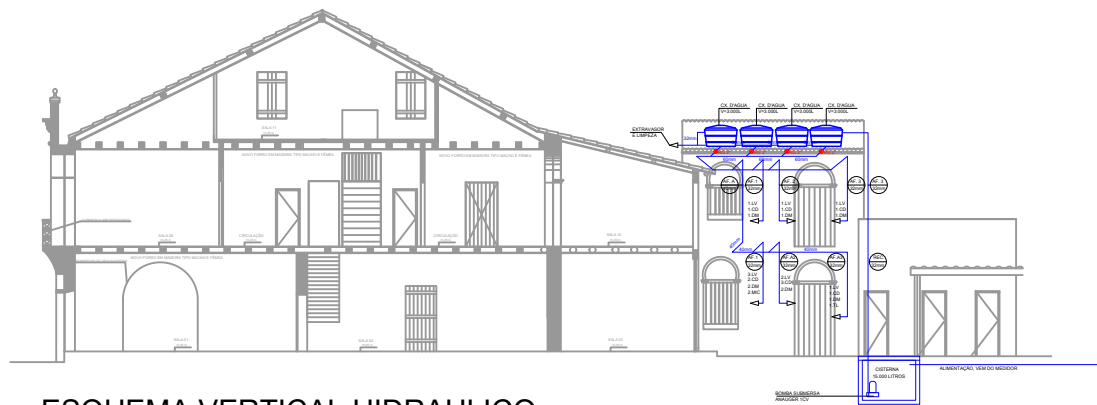
ESQUEMA VERTICAL HIDRAULICO ESCALA 1/200
