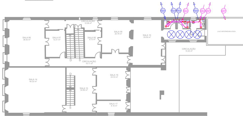
PLANTA BAIXA 1º PAVIMENTO / HIDROSSANITARIO ESCALA 1/200
