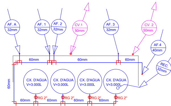
PLANTA CAIXAS D'ÁGUA ESCALA 1/75
