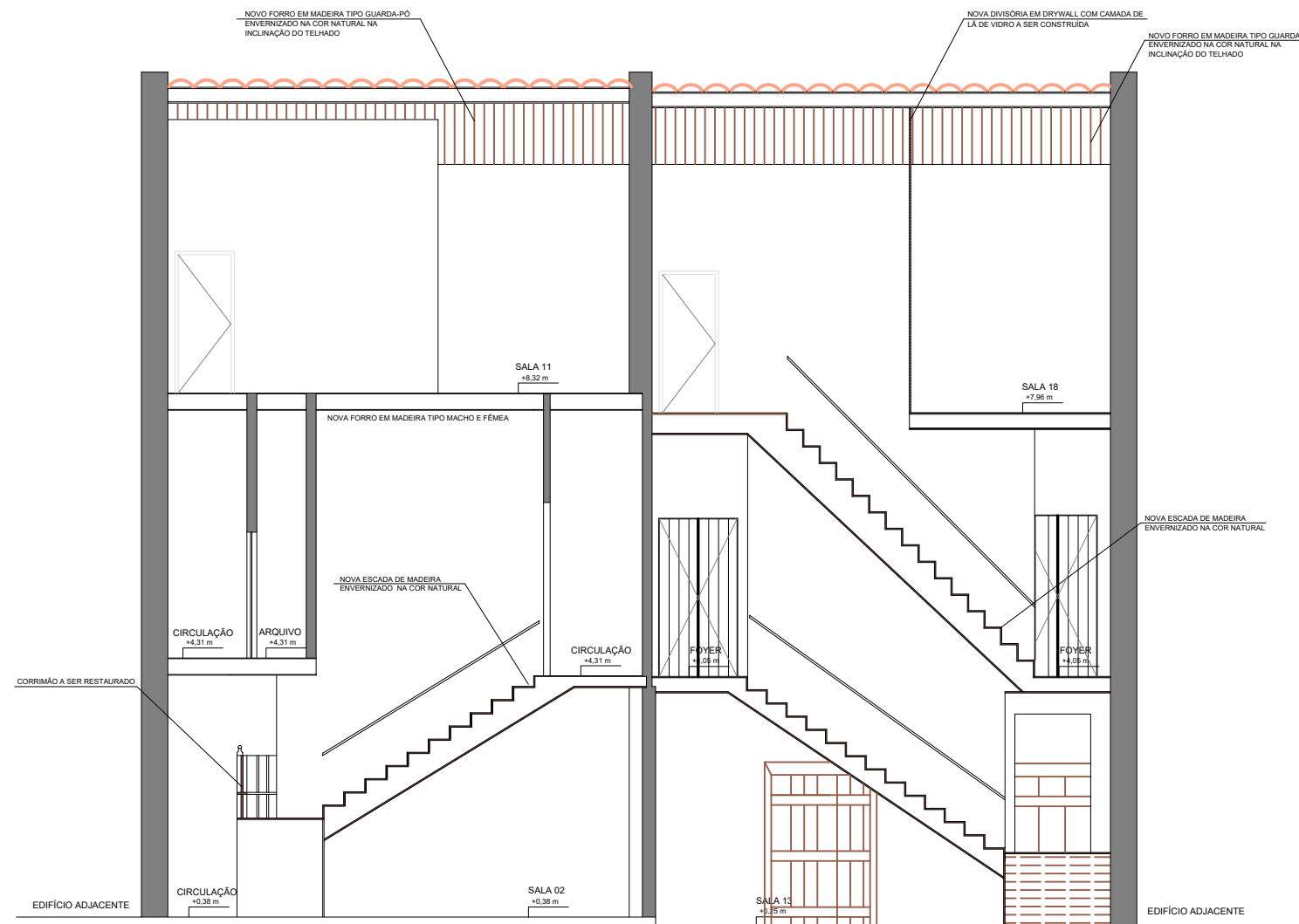
01 CORTE CC ESCALA 1/125
