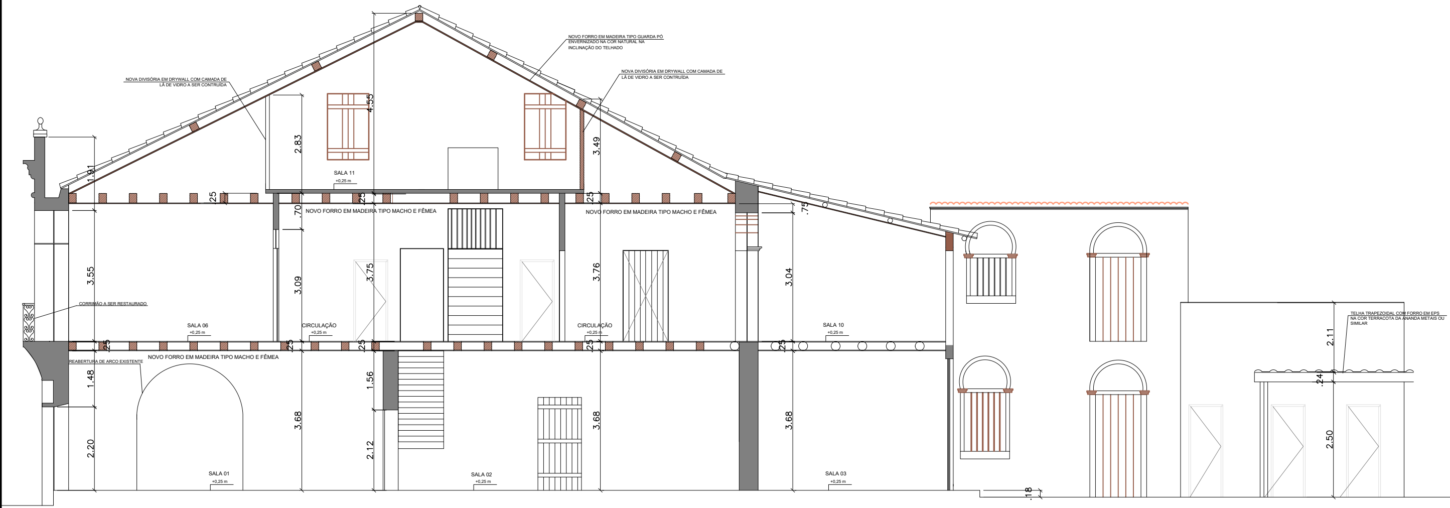
01 CORTE AA ESCALA 1/125
