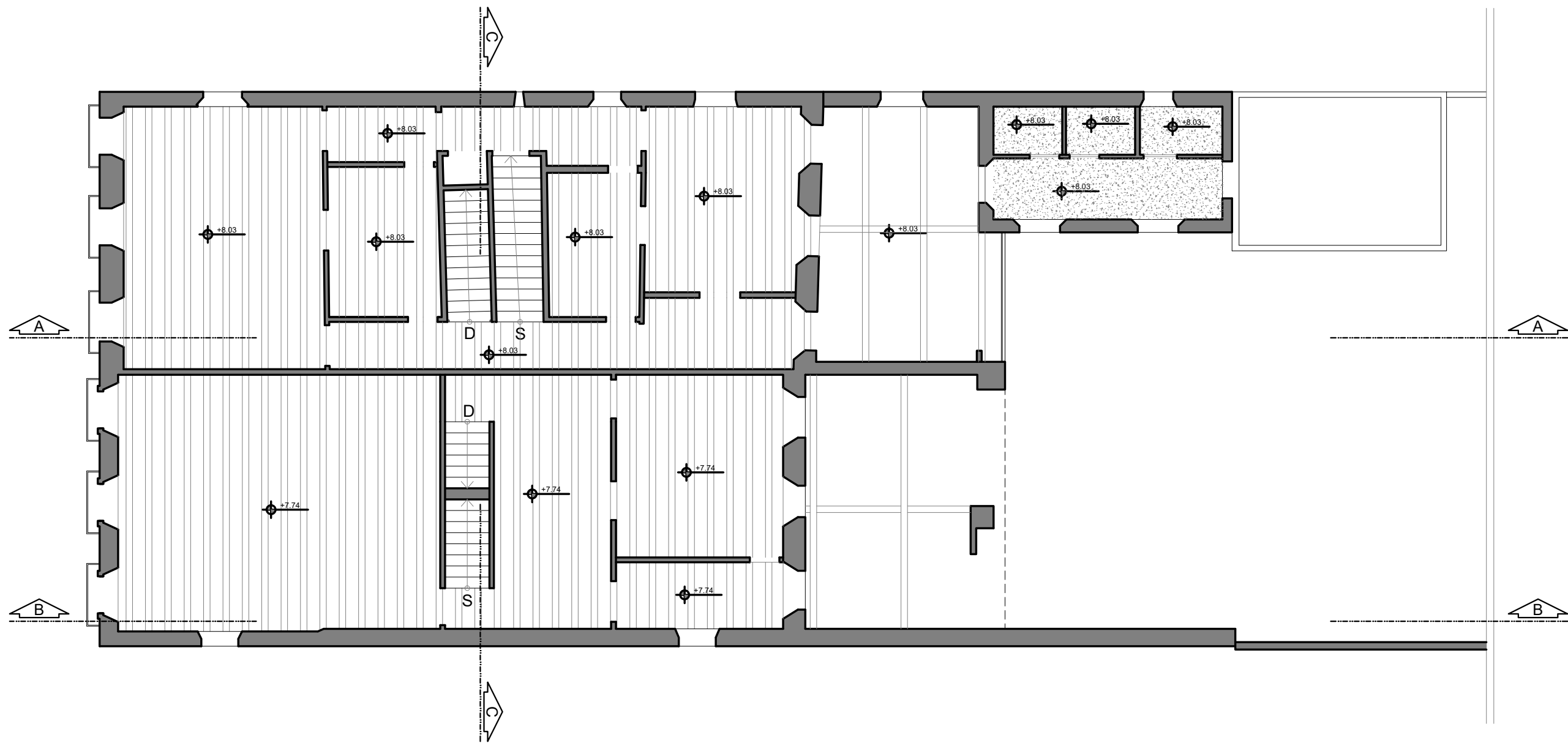
01 PLANTA DE FORRO - PRIMEIRO PAVIMENTO ESCALA 1/125
