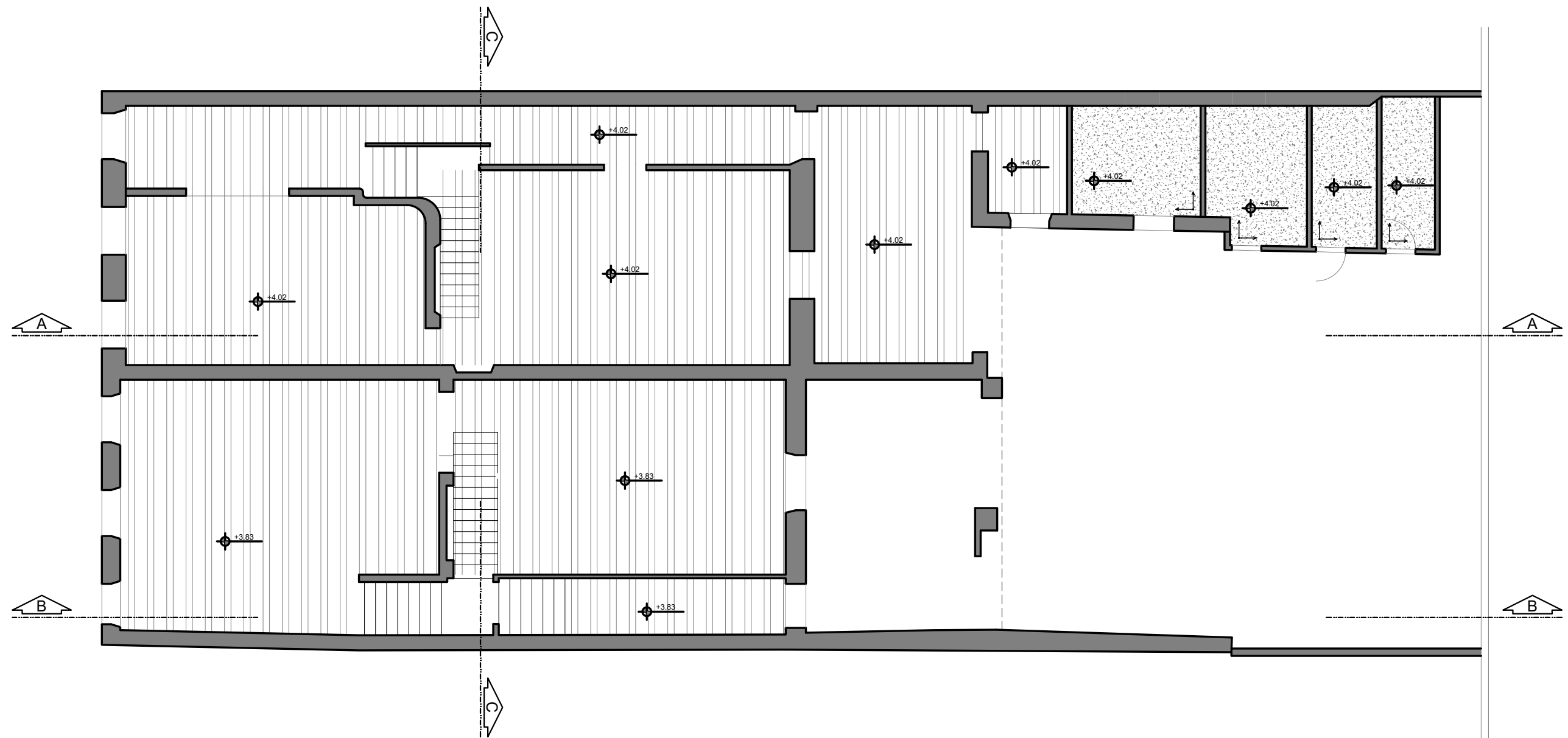
01 PLANTA DE FORRO - TÉRREO ESCALA 1/125
