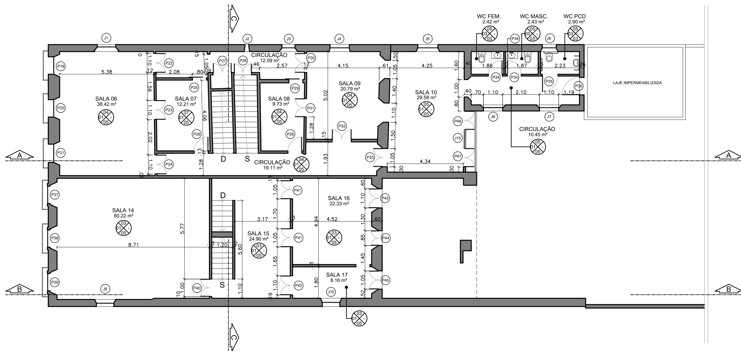
01 PLANTA BAIXA - PRIMEIRO PAVIMENTO ESCALA 1/125
