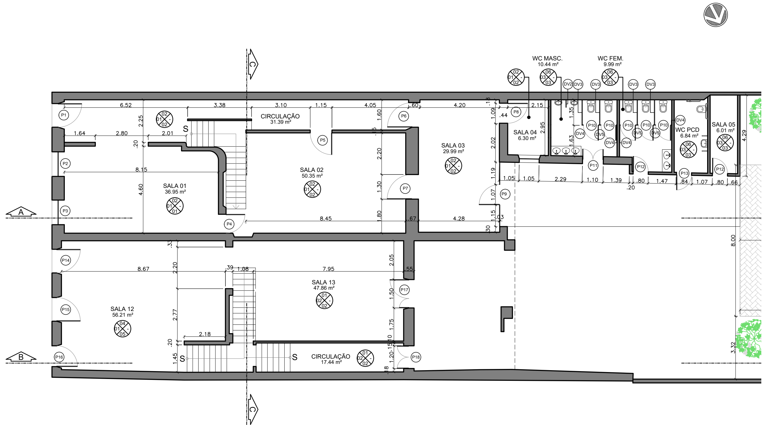
01 PLANTA BAIXA - TÉRREO PARTE 01 ESCALA 1/125
