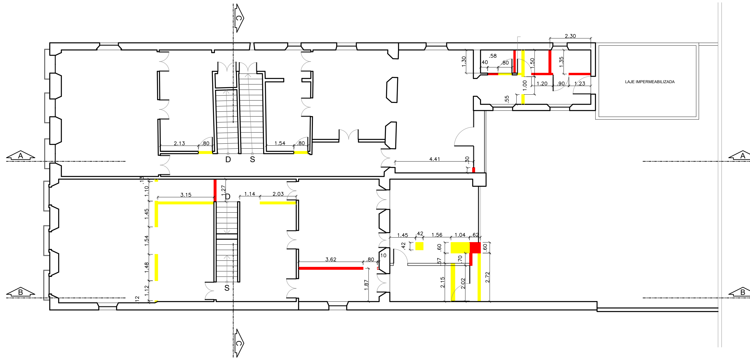
02 PLANTA BAIXA - PRIMEIRO PAVIMENTO ESCALA 1/125
