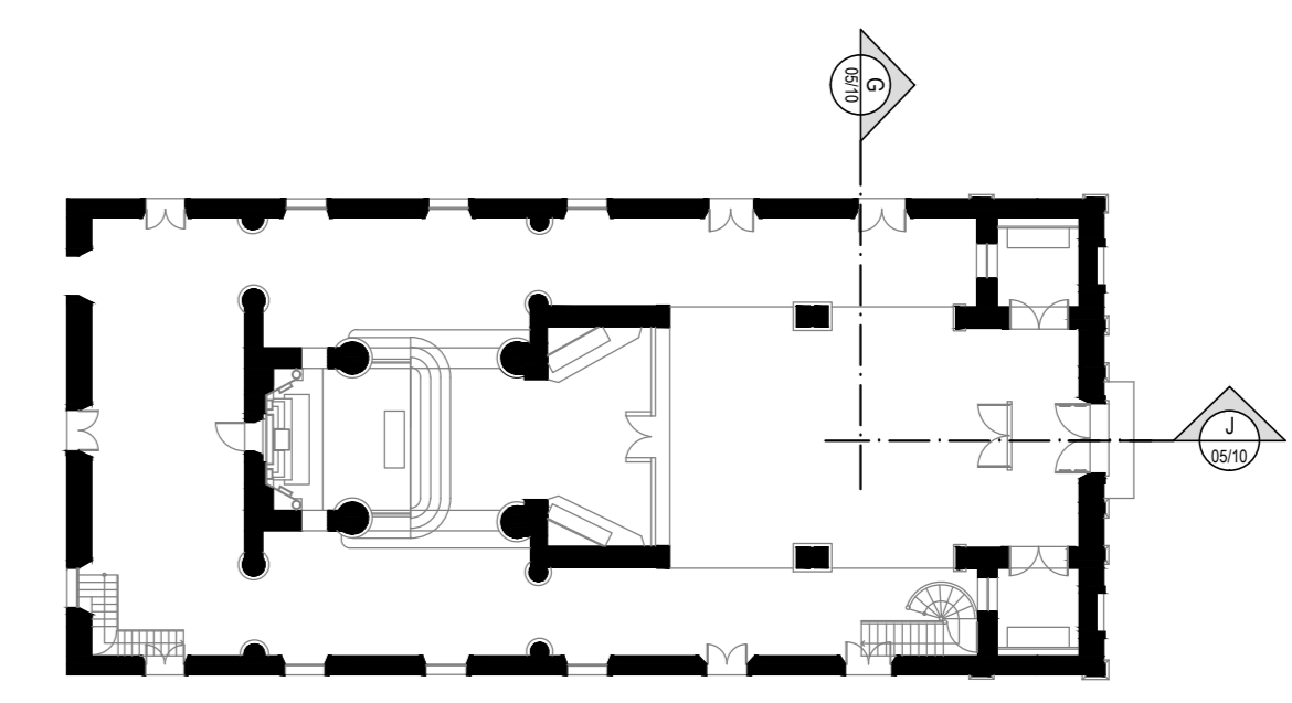
03 PLANTA INDICATIVA DE CORTE ESC. 1/200
