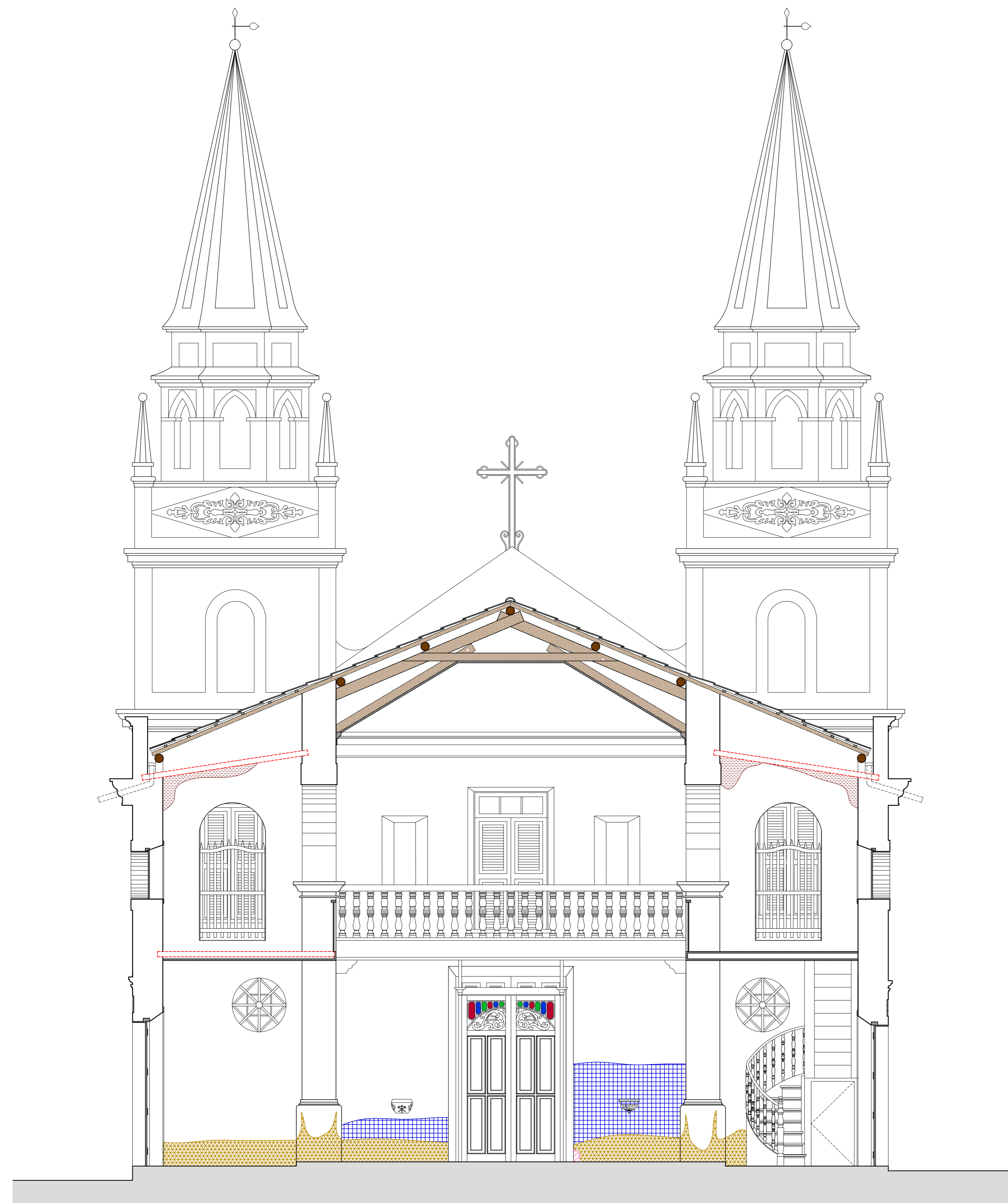
01 CORTE G ESC. 1/50
