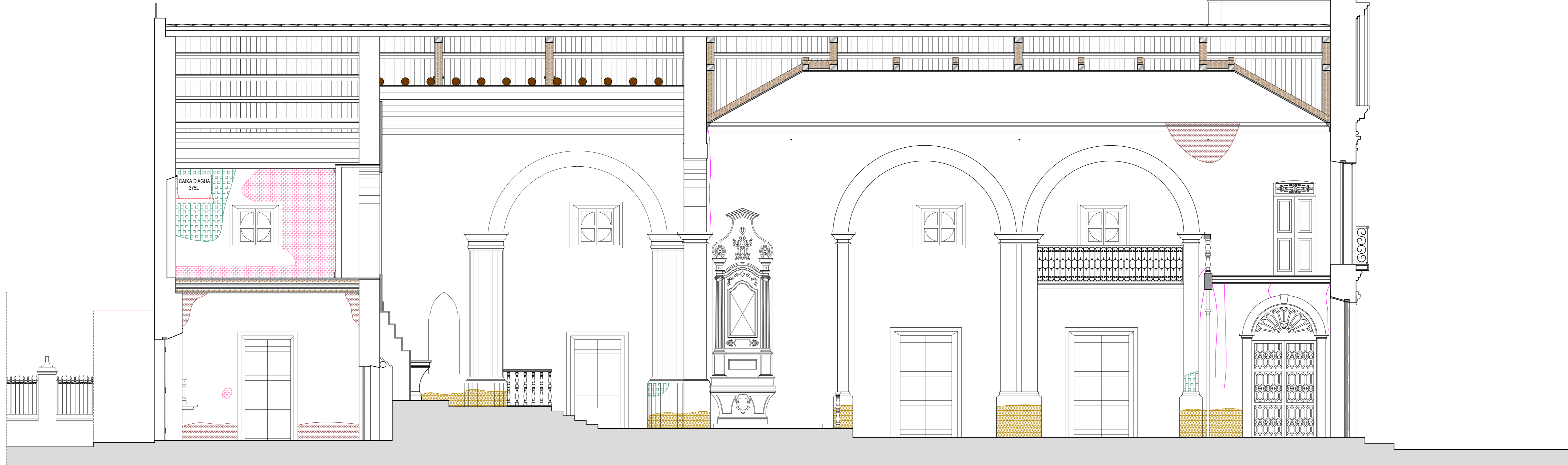
02 CORTE J ESC. 1/50
