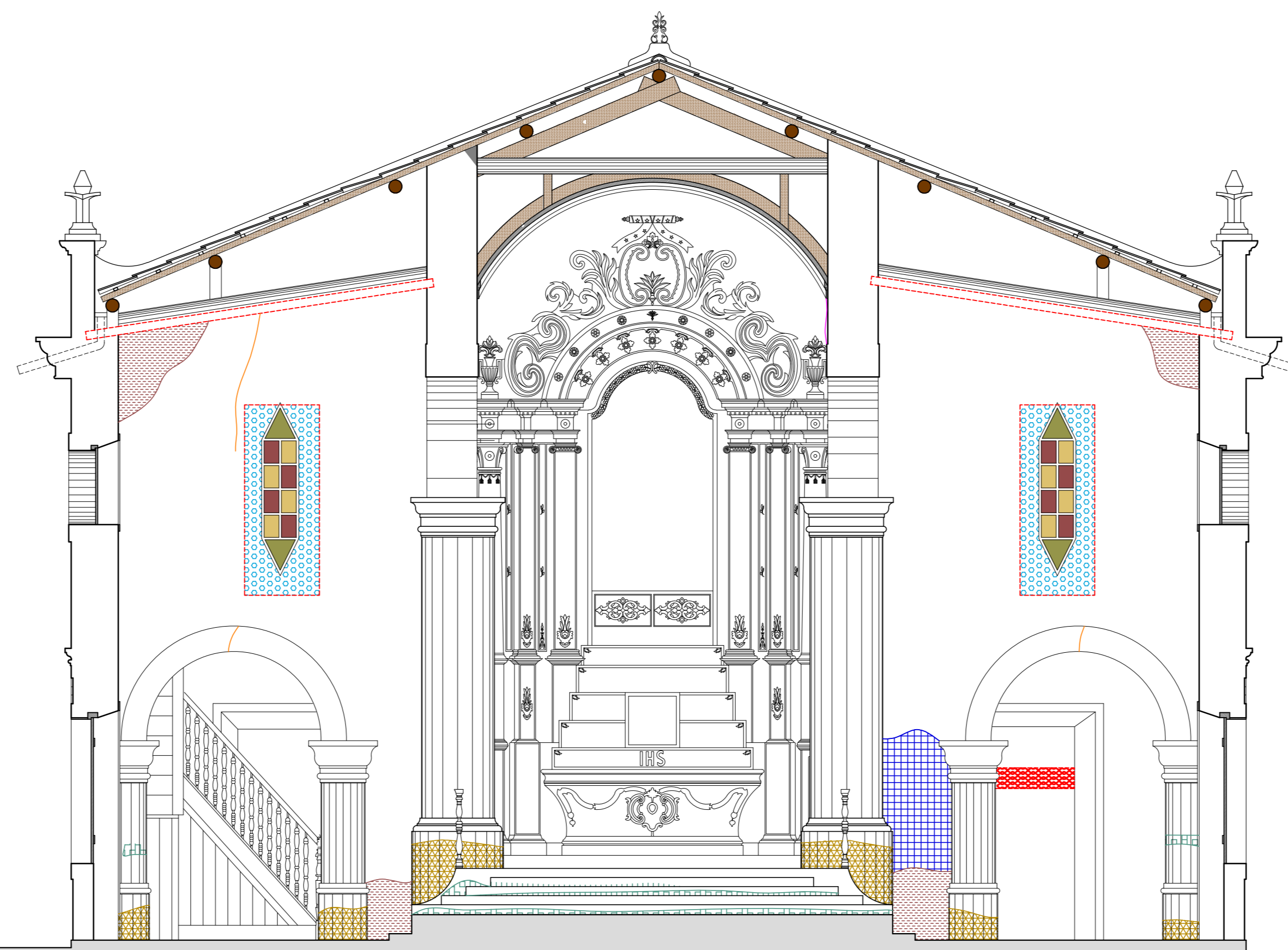
02 CORTE B ESC. 1/50
