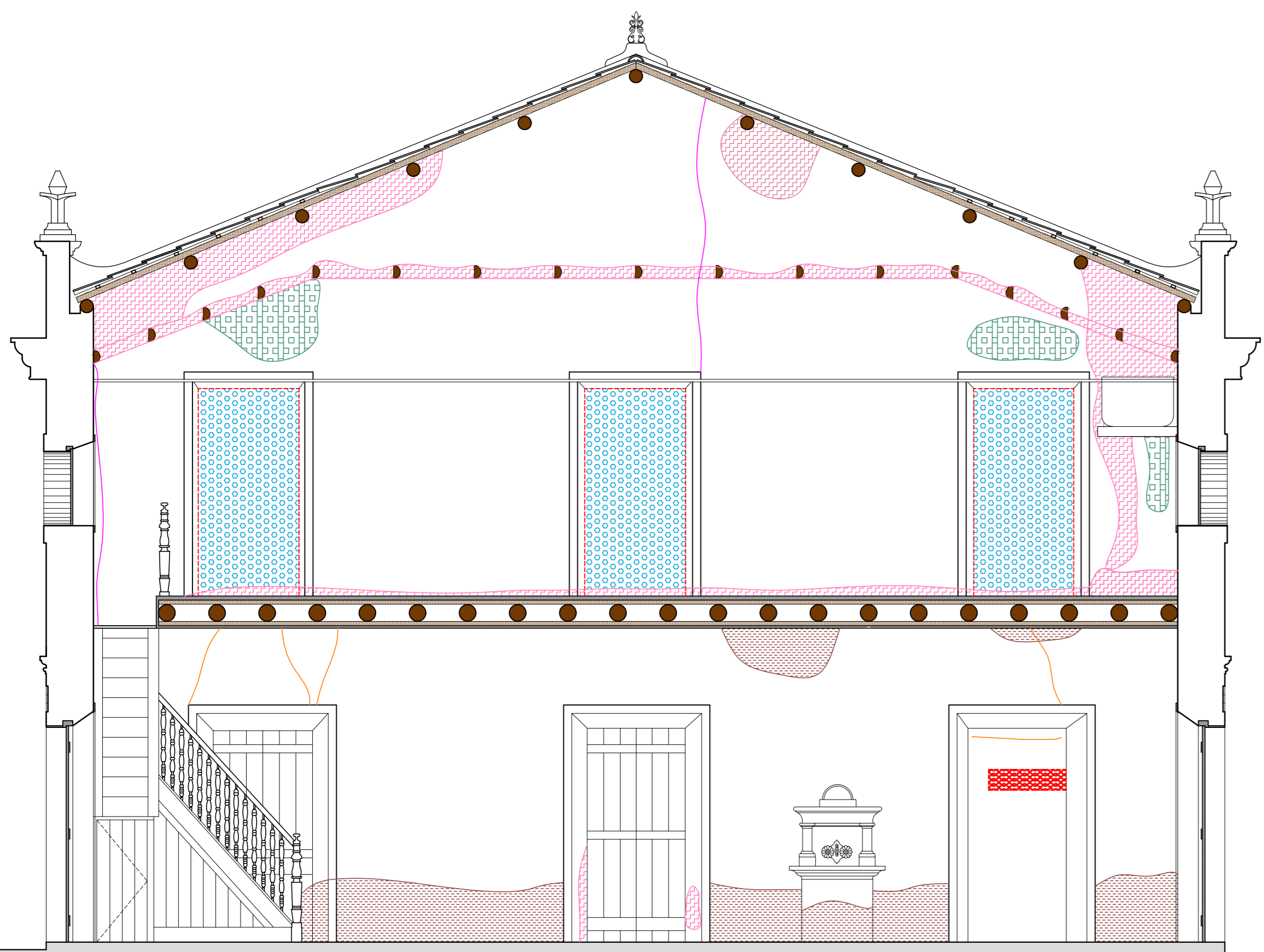
01 CORTE A ESC. 1/50
