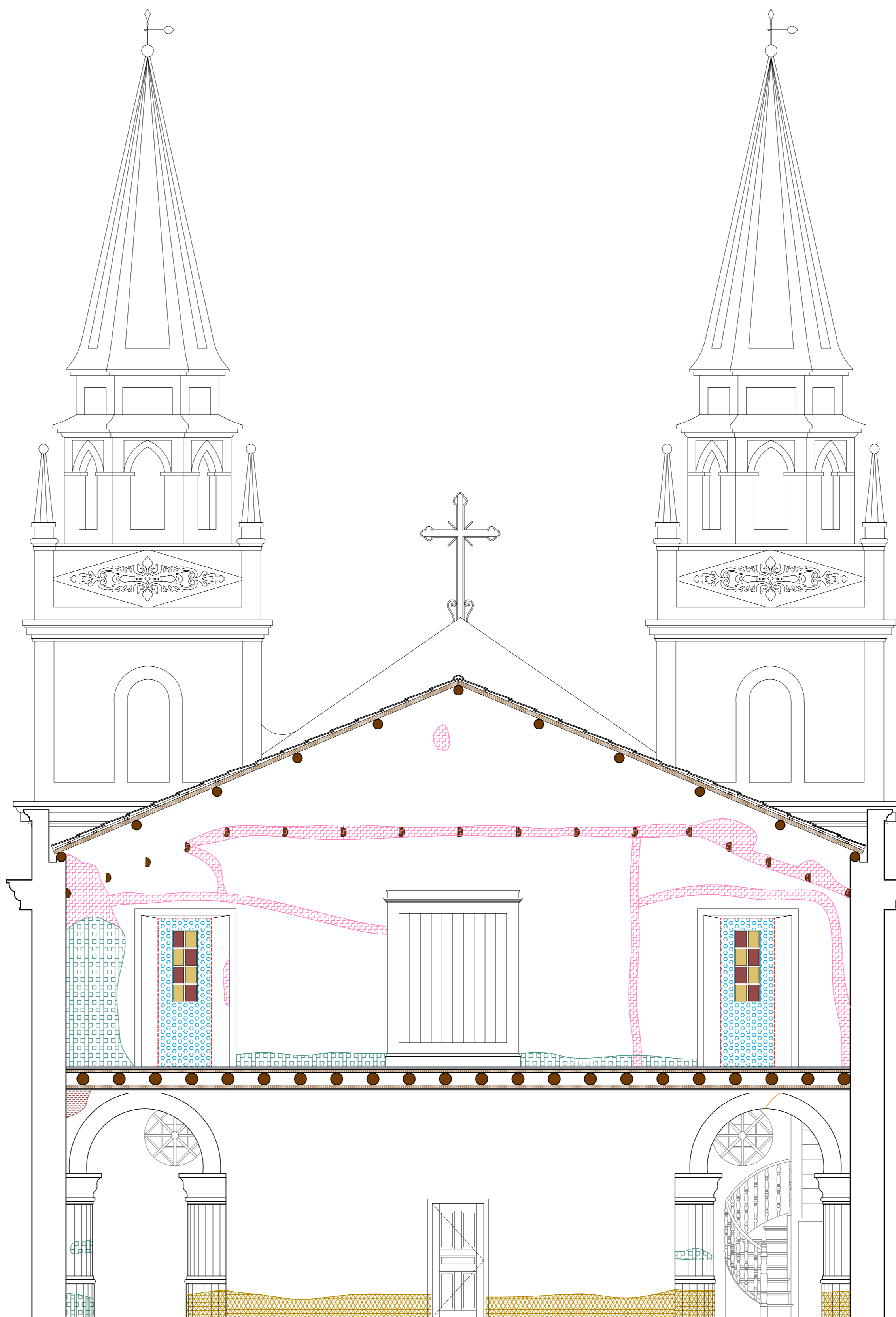
05 CORTE E ESC. 1/50
