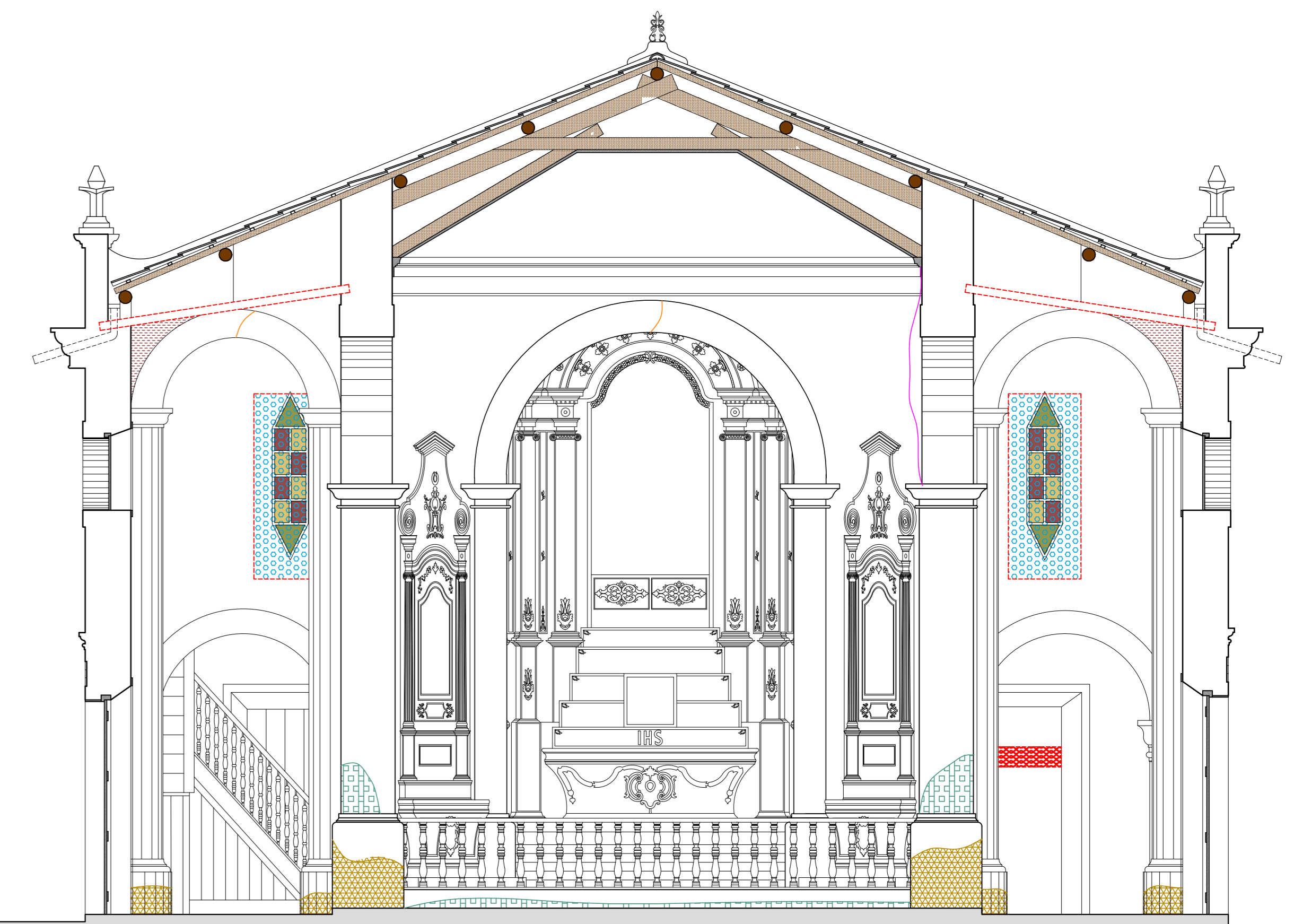
03 CORTE C ESC. 1/50
