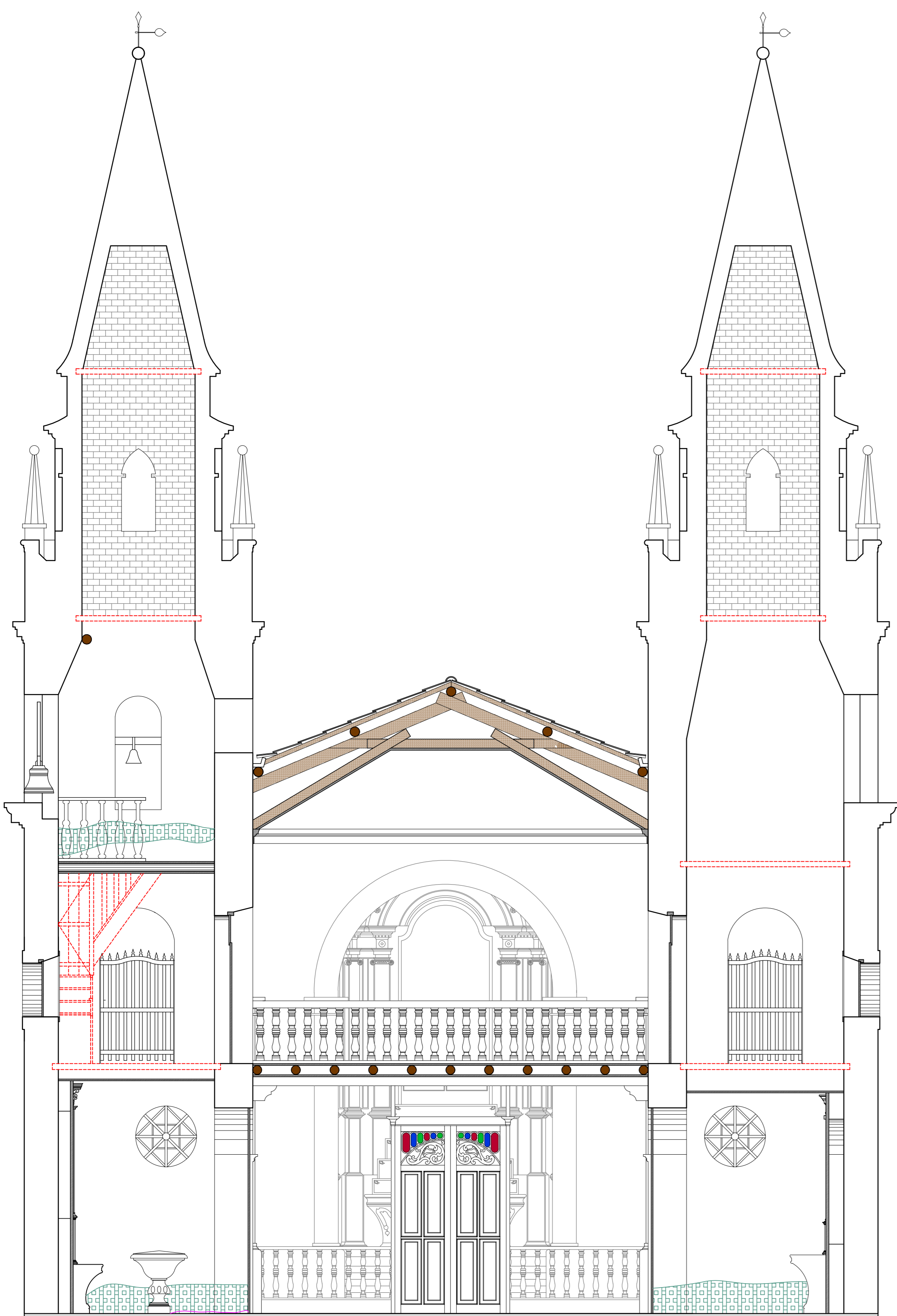
04 CORTE D ESC. 1/50
