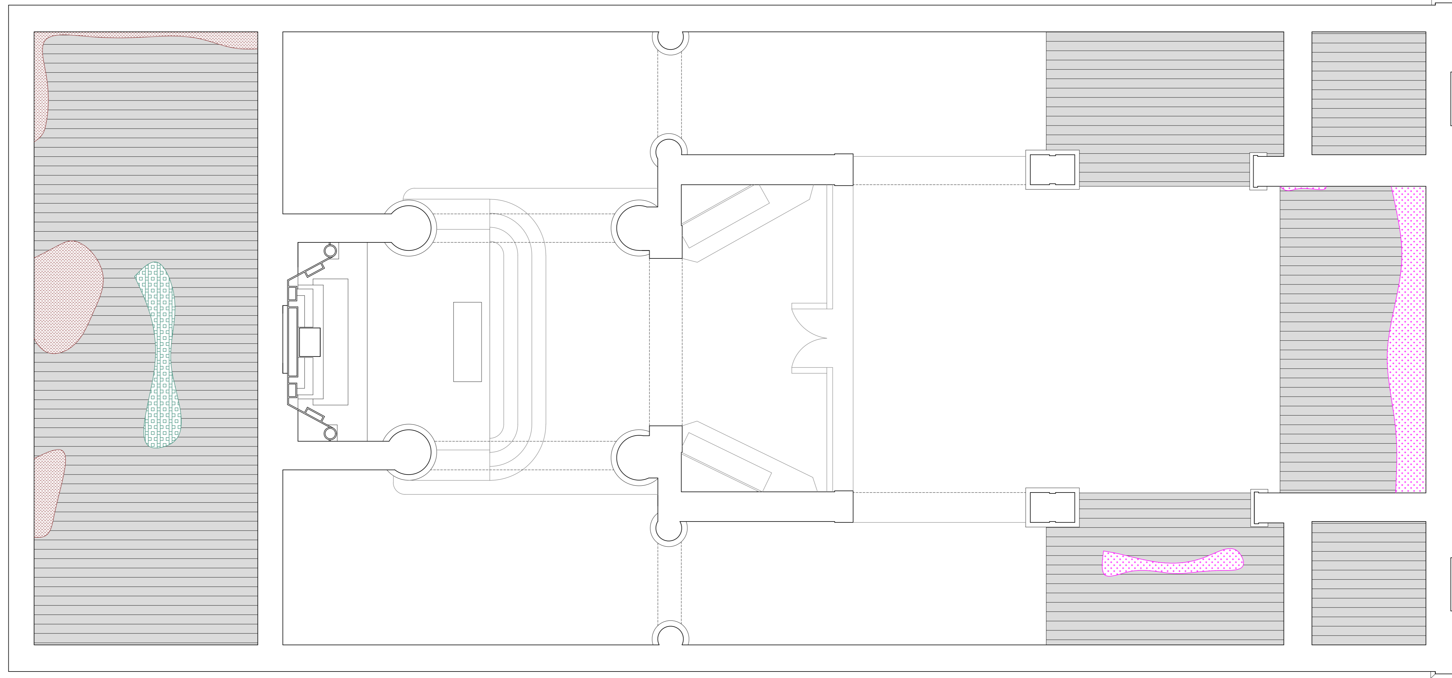
01 PLANTA DE FORRO PAV. TÉRREO ESC. 1/50
