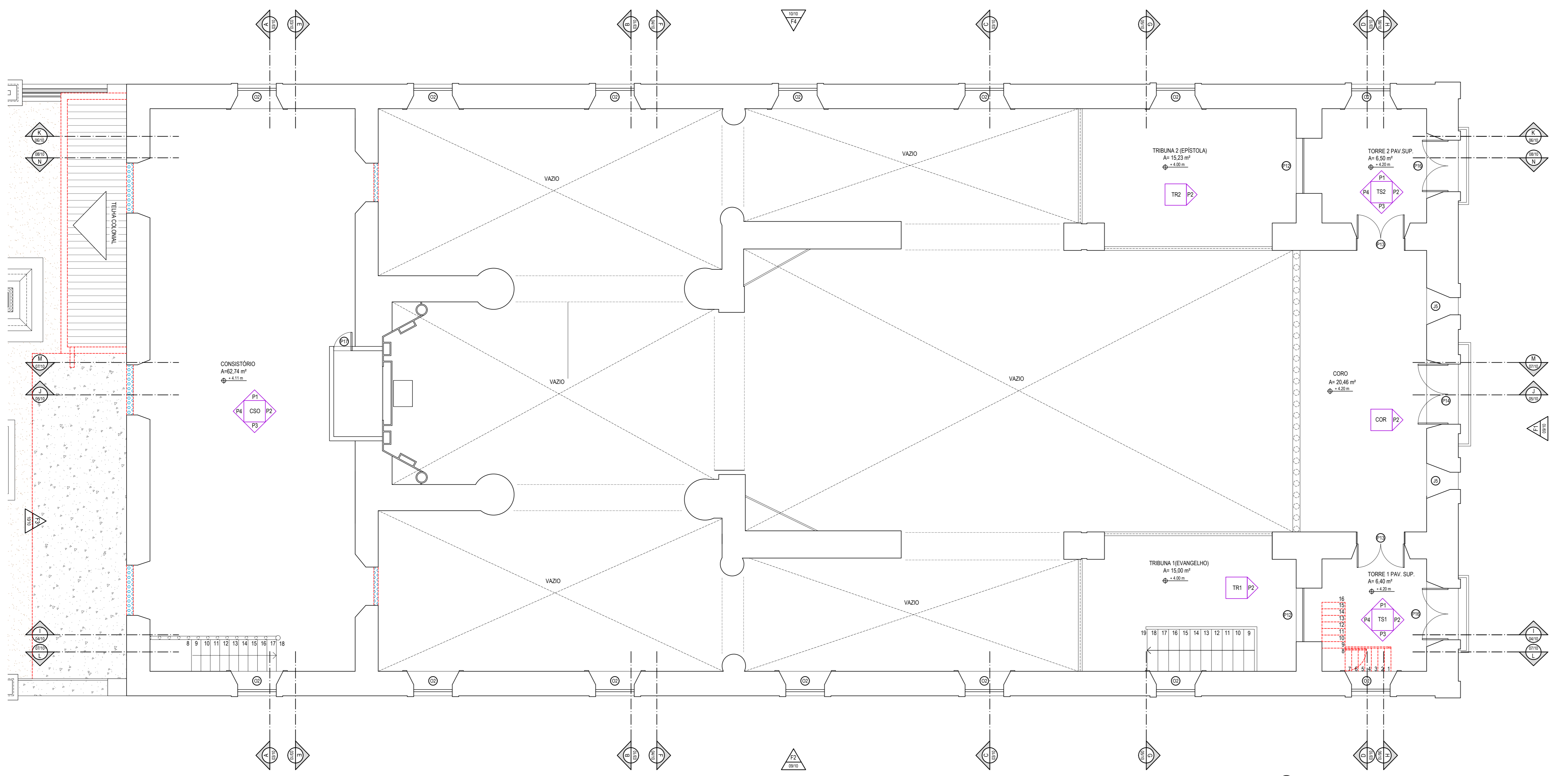
02 PLANTA DE REFORMA PAV. SUPERIOR ESC. 1/50
