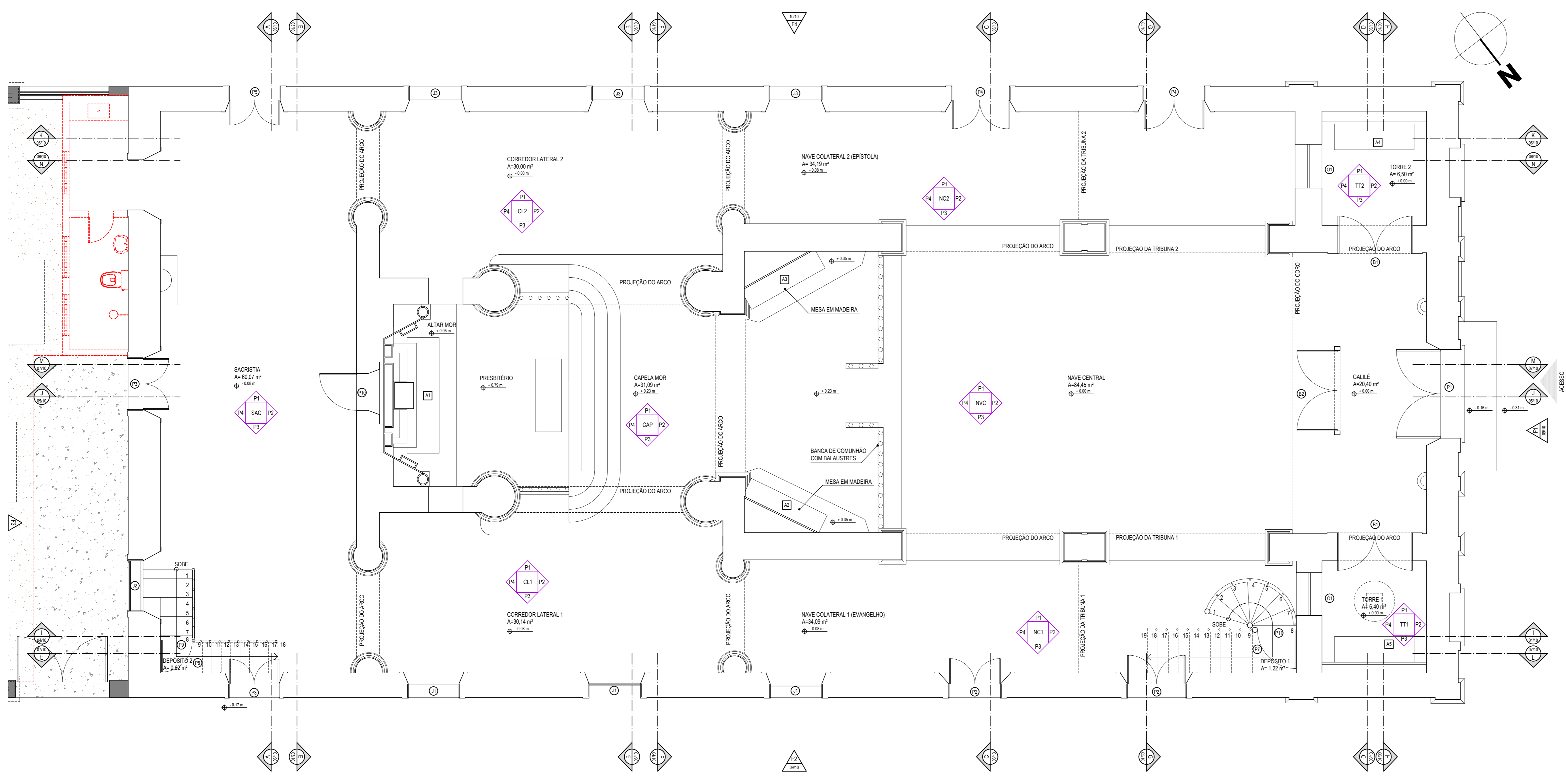
01 PLANTA DE REFORMA TÉRREO ESC. 1/50
