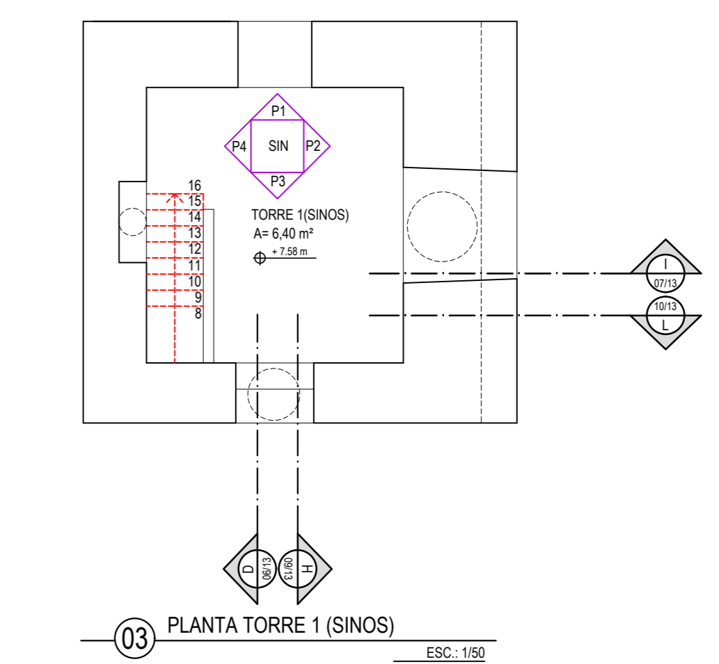
03 PLANTA TORRE 1 (SINOS) ESC. 1/50
