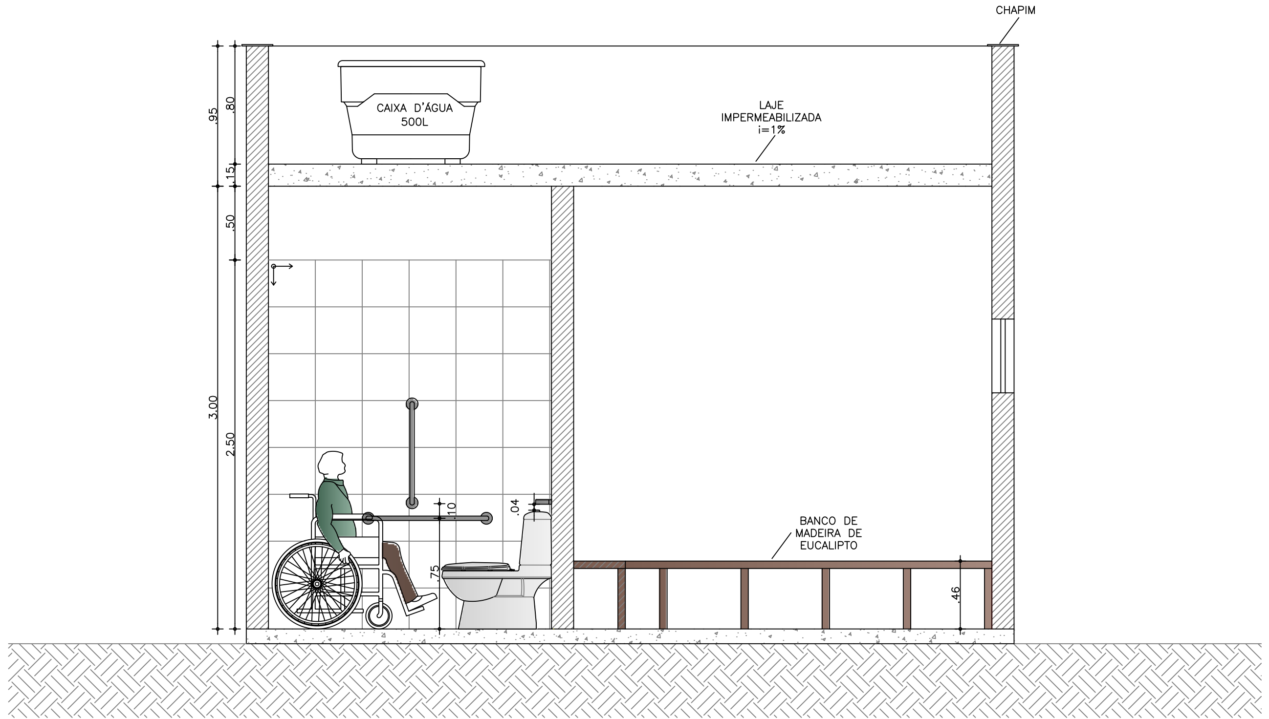
1 CORTE AA' ESCALA 1/25
