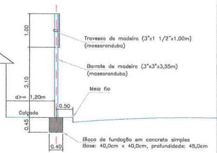
DETALHE DO SUPORTE DE MADEIRA 8x8cm A SER UTILIZADO PARA FIXAÇÃO DAS PLACAS TIPO B Escala 1/50
