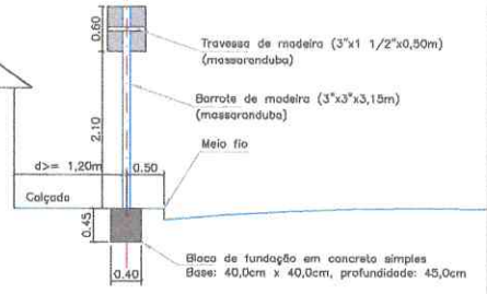
DETALHE DO SUPORTE MADEIRA 8x8cm A SER UTILIZADO PARA FIXAÇÃO DAS PLACAS TIPO A Escala 1/50
