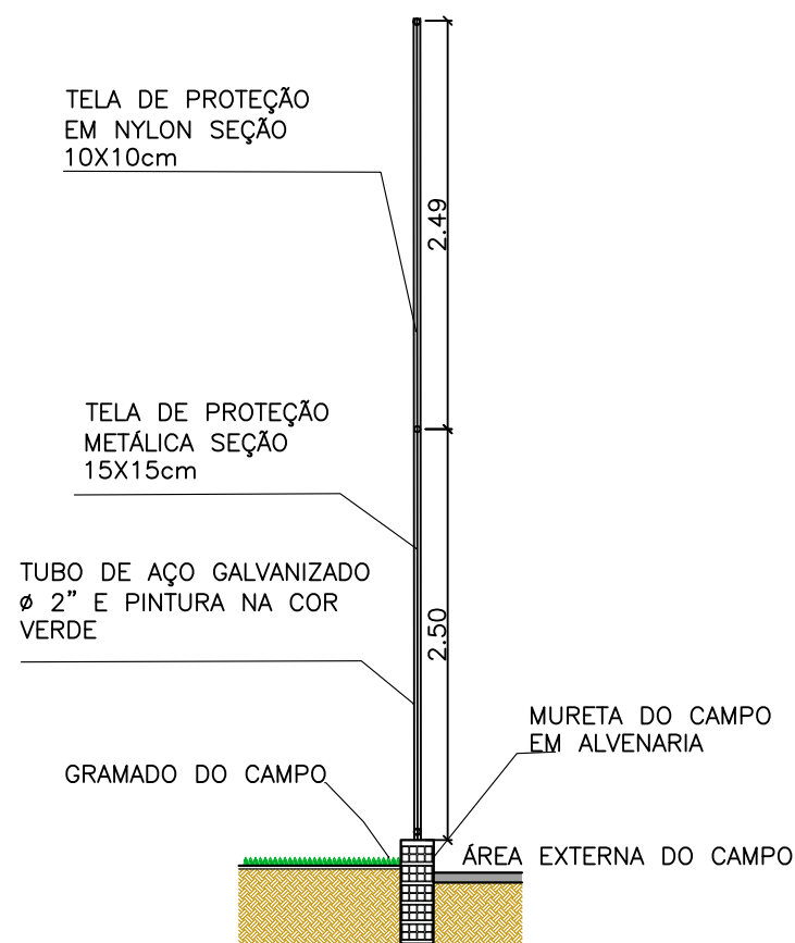
CORTE esc 1:75
