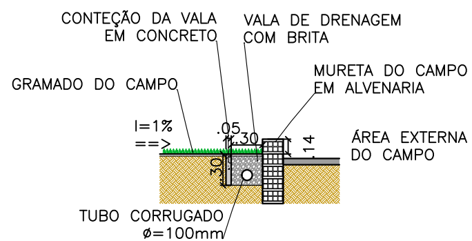
DETALHE 02 esc 1:75
