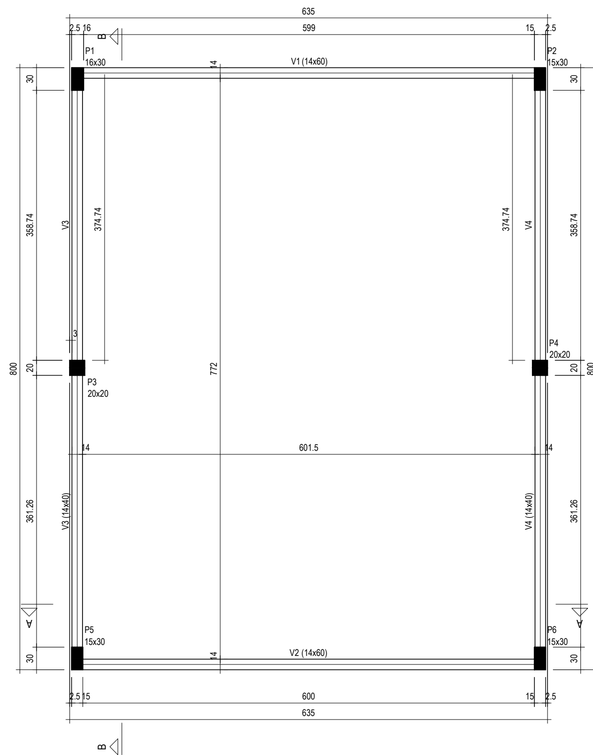
FORMA DO PAVIMENTO SUPERIOR (NÍVEL 320) ESC: 1:50
