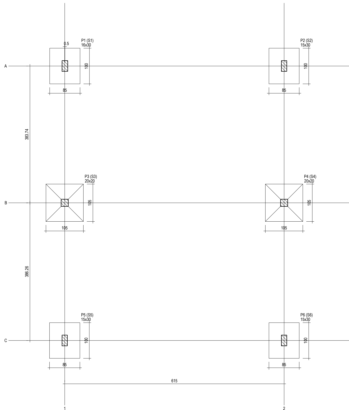
PLANTA DE LOCAÇÃO ESC: 1:50
