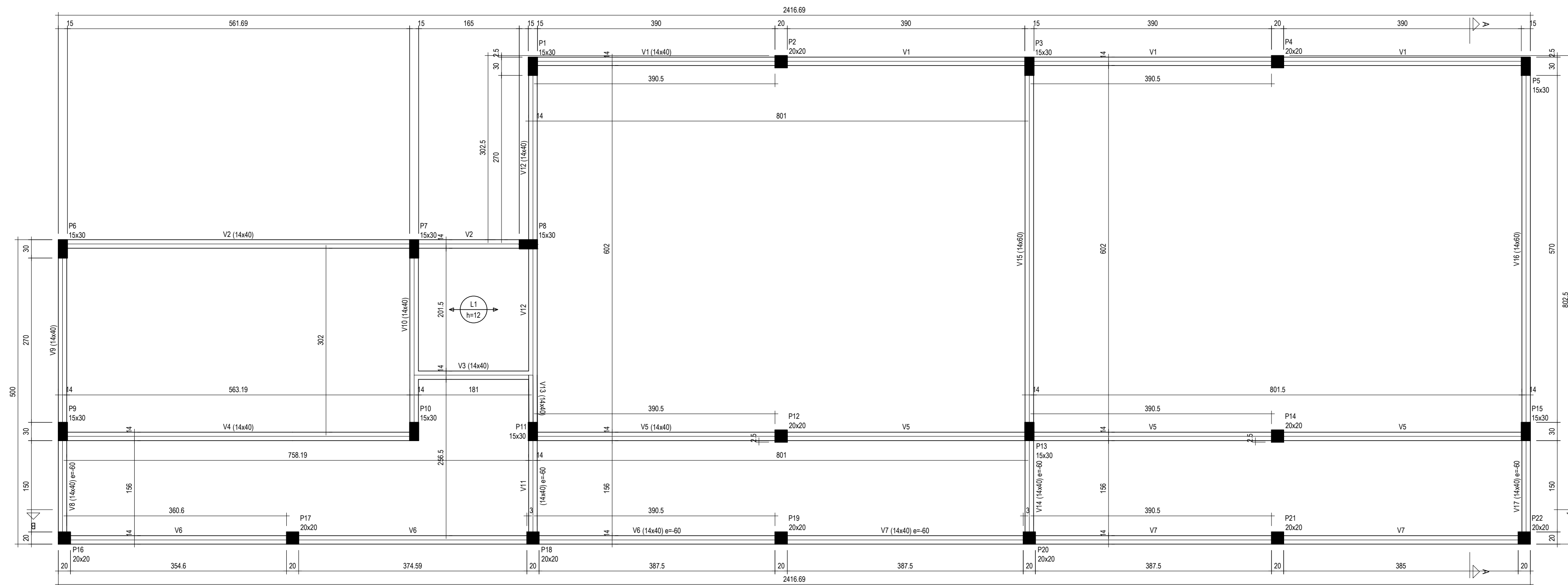
FORMA DO PAVIMENTO SUPERIOR (NÍVEL 320) ESC: 1/50
