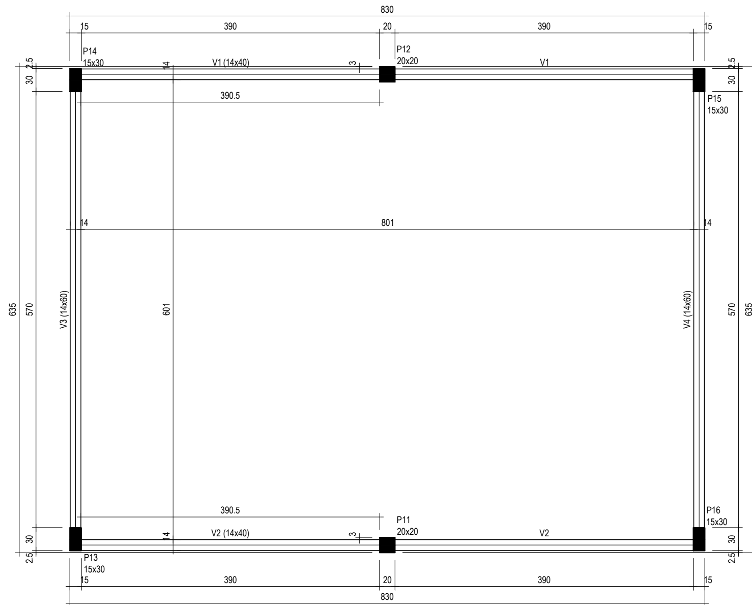
FORMA DO PAVIMENTO SUPERIOR (NÍVEL 320) ESC: 1:50
