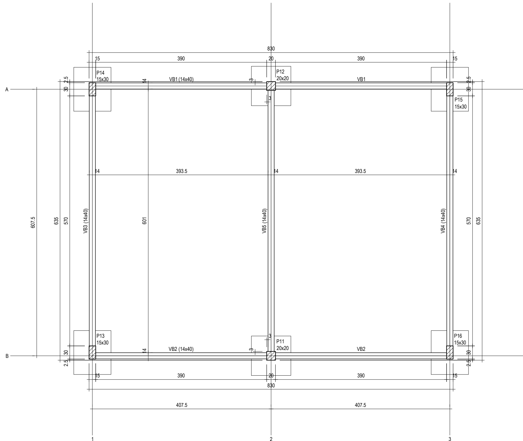
FORMA DO PAVIMENTO TÉRREO (NÍVEL 0) ESC: 1:50
