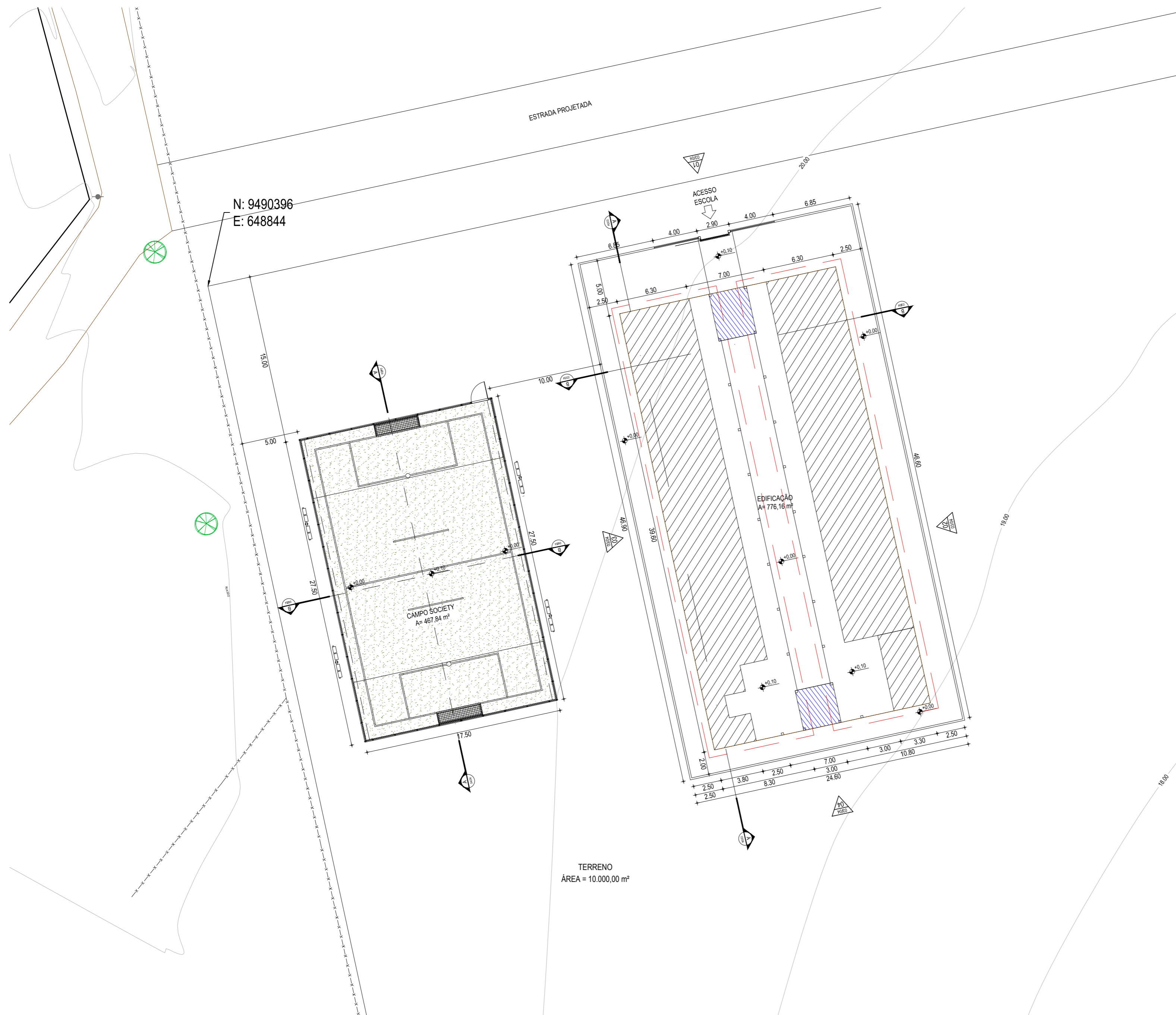
01 PLANTA DE IMPLANTAÇÃO ESCALA: 1/250
