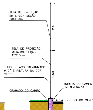
CORTE esc 1:75
