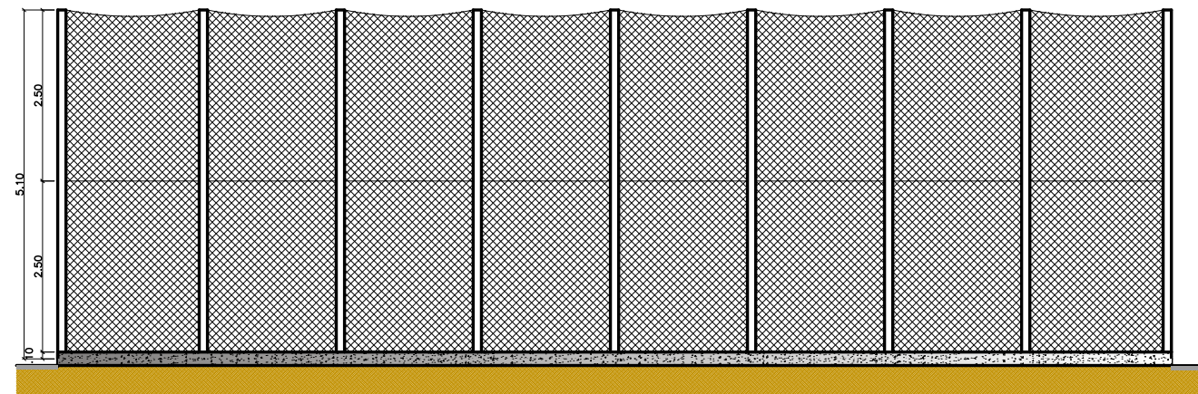
VISTA 01 esc 1:75
