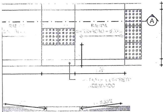
05 | DETALHE 05 - RAMPA ACESSIVEL Esc: 1/50
