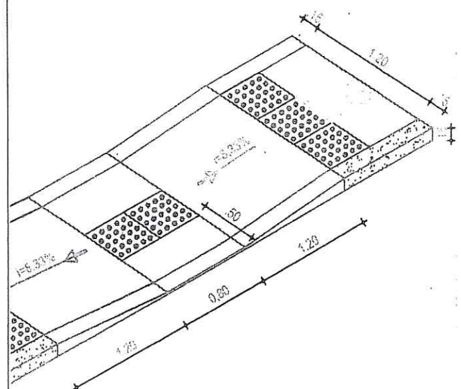
05 | DETALHE 05 - RAMPA ACESSIVEL Esc: 1/50
