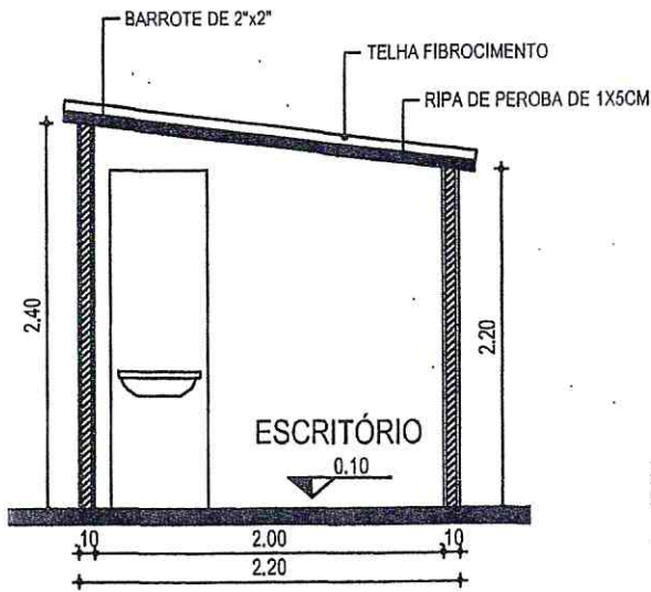
01 | CORTE B B ESC.: 1/50
