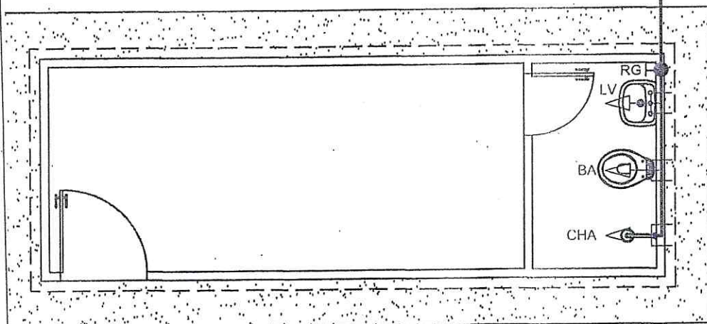
1 | PLANTA DE INST. HIDRAULICA ESC.: 1/50
