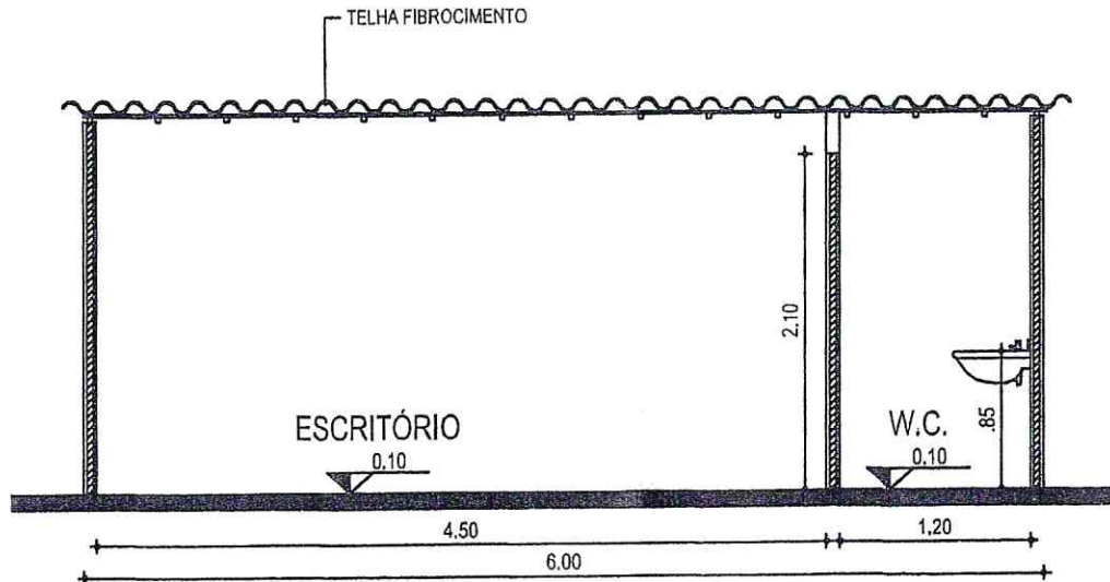
01 | CORTE A A ESC.: 1/50
