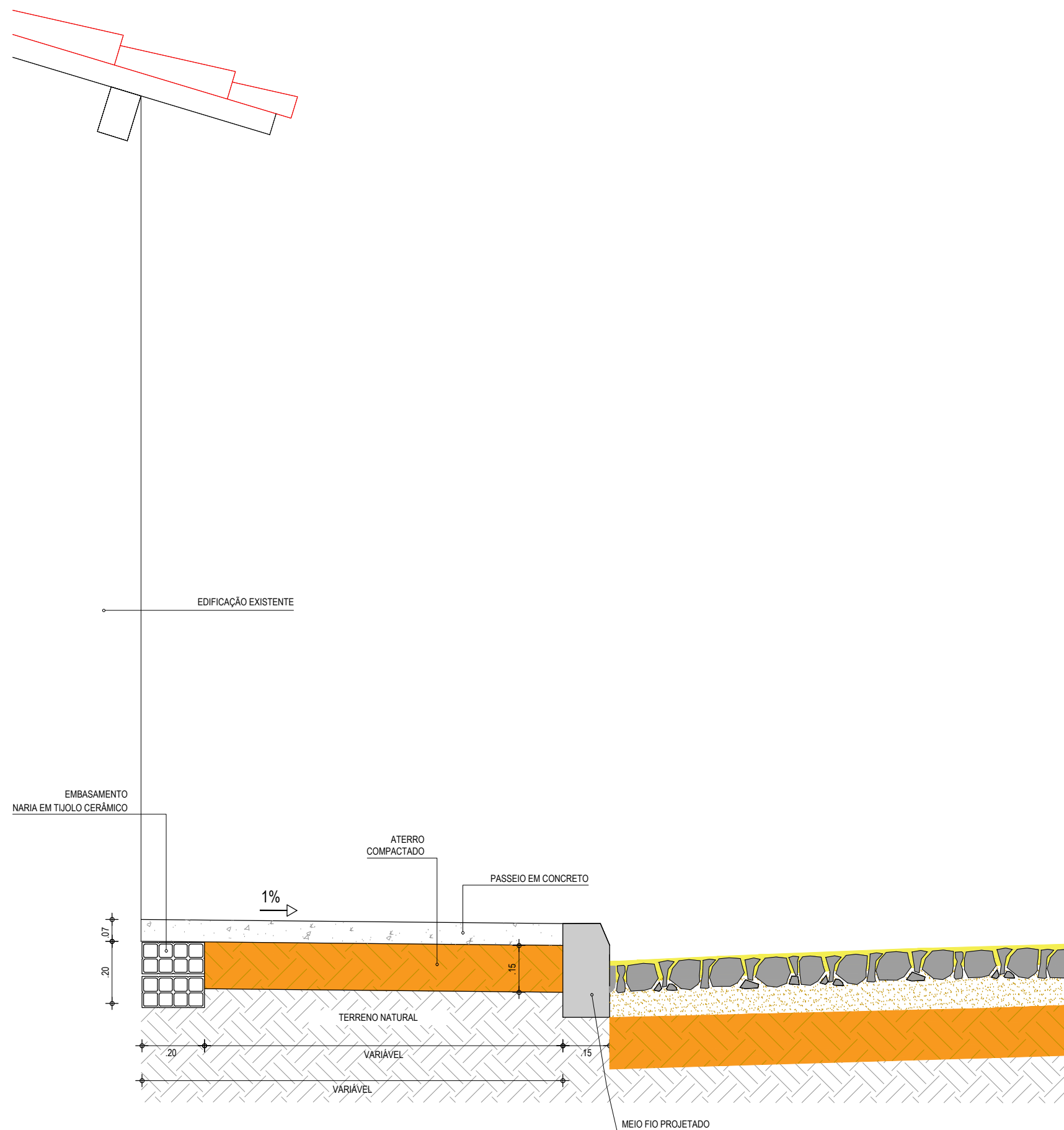
01 DETALHE DO PASSEIO ESCALA: SEM
