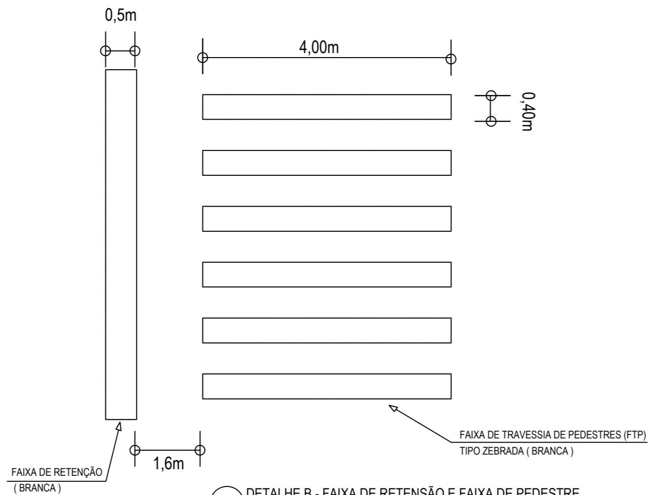
03 DETALHE B - FAIXA DE RETENÇÃO E FAIXA DE PEDESTRE ESCALA: SEM
