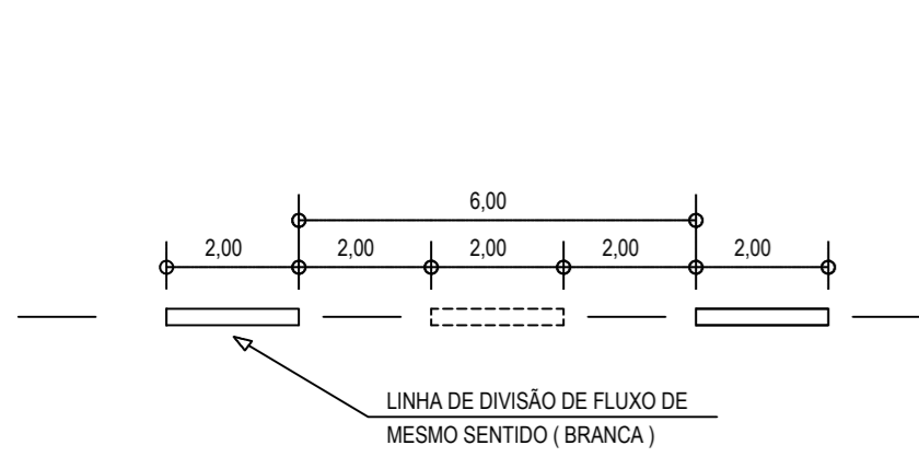
02 DETALHE A - LINHAS DEMARCADORAS DE FAIXA ESCALA: SEM
