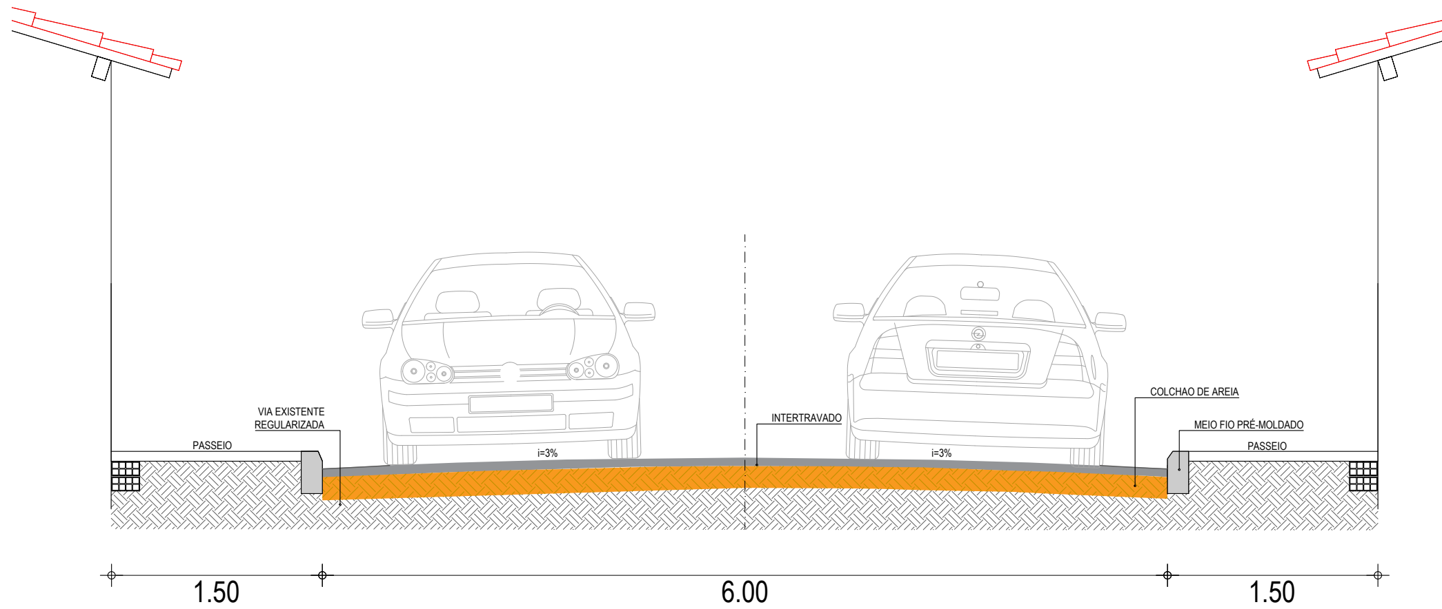
01 SEÇÃO TIPO SEM ESCALA
