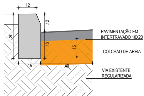
02 DETALHE DOS MATERIAS SEM ESCALA
