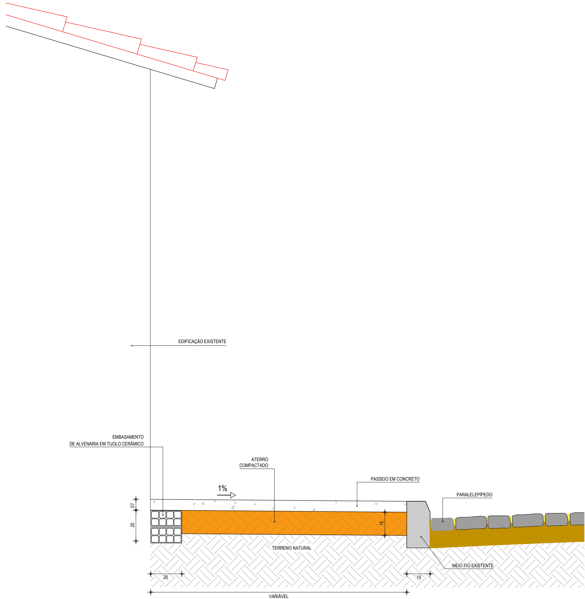
01 DETALHE DO PASSEIO ESCALA: 1/15
